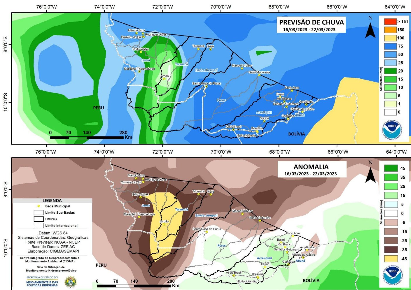
Figura 2: Prognóstico NCEP-GFS/USA.
