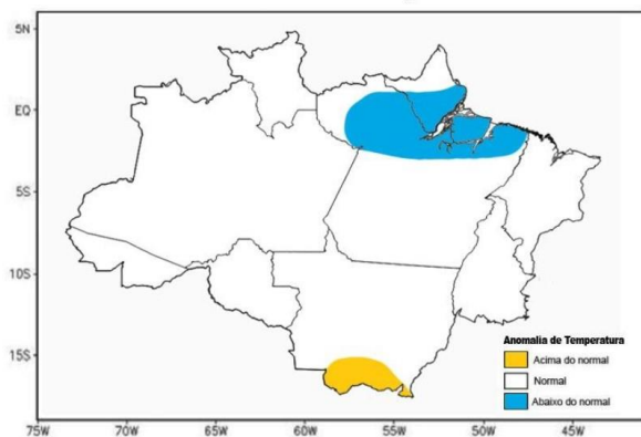
Figura 03 - Prognóstico de anomalias de temperatura para o trimestre Fevereiro-Março-Abril/2023.
