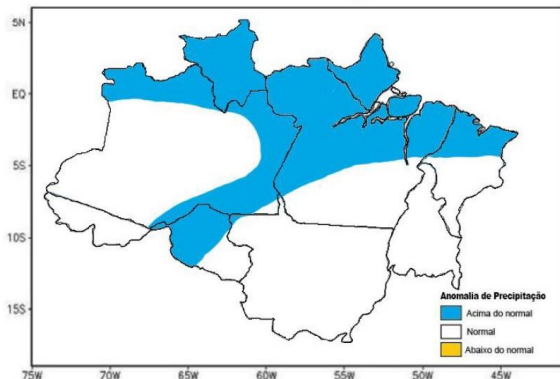
Figura 02 - Prognóstico de anomalias de precipitação para o trimestre Fevereiro-Março-Abril/2023.
