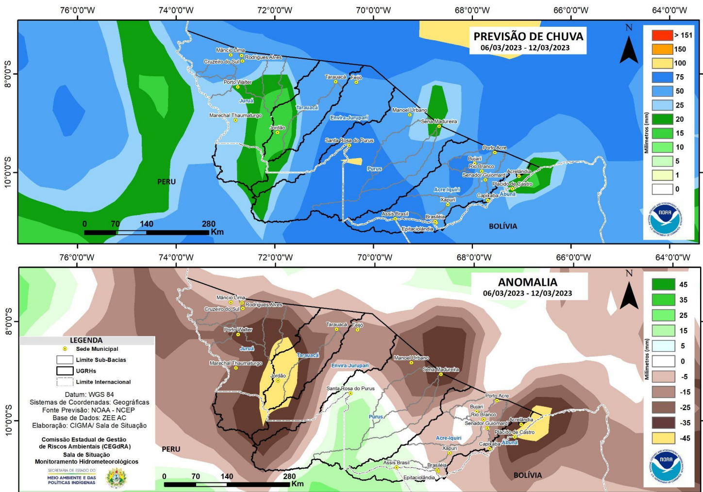
Figura 2: Prognóstico NCEP-GFS/USA.
