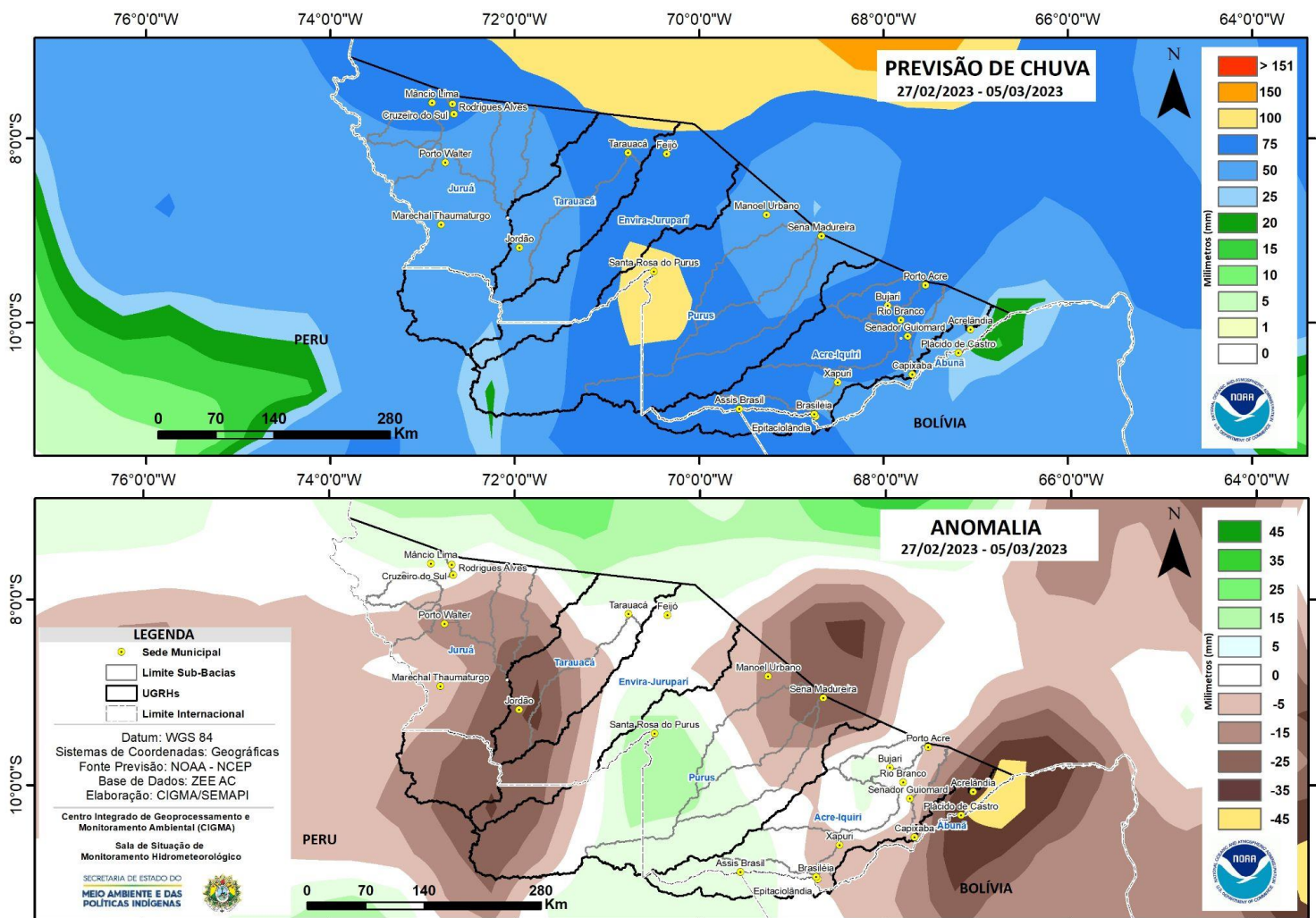
Figura 2: Prognóstico NCEP-GFS/USA.
