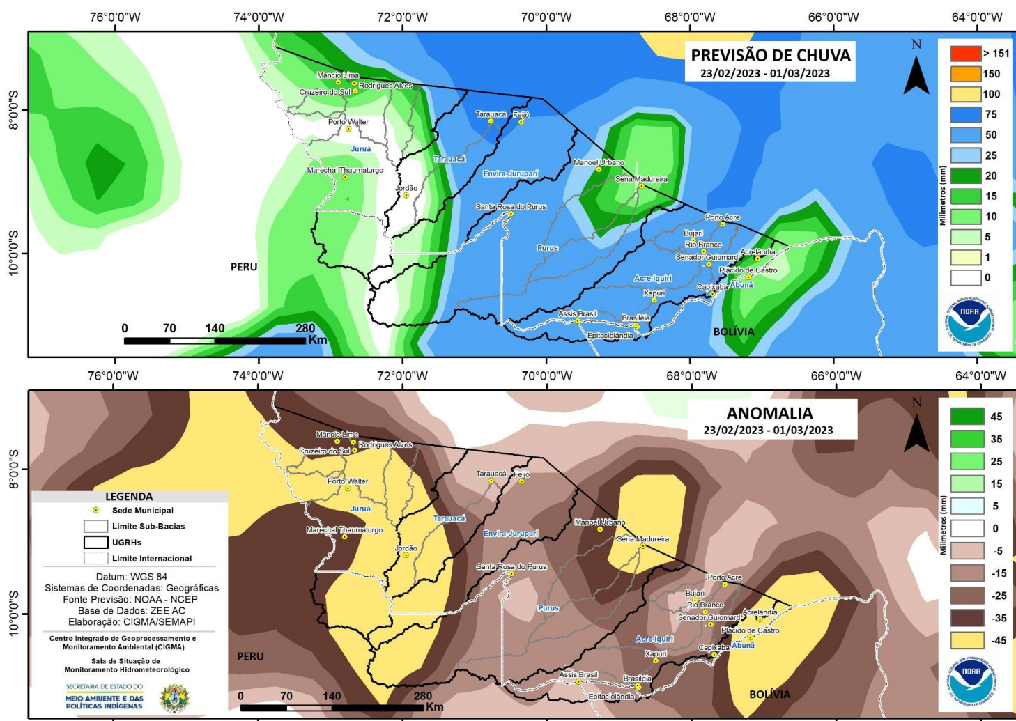
Figura 2: Prognóstico NCEP-GFS/USA.
