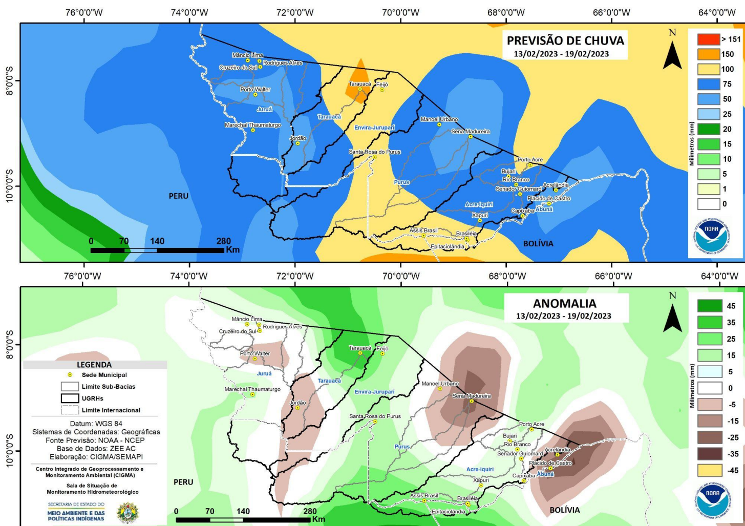
Figura 2: Prognóstico NCEP-GFS/USA.
