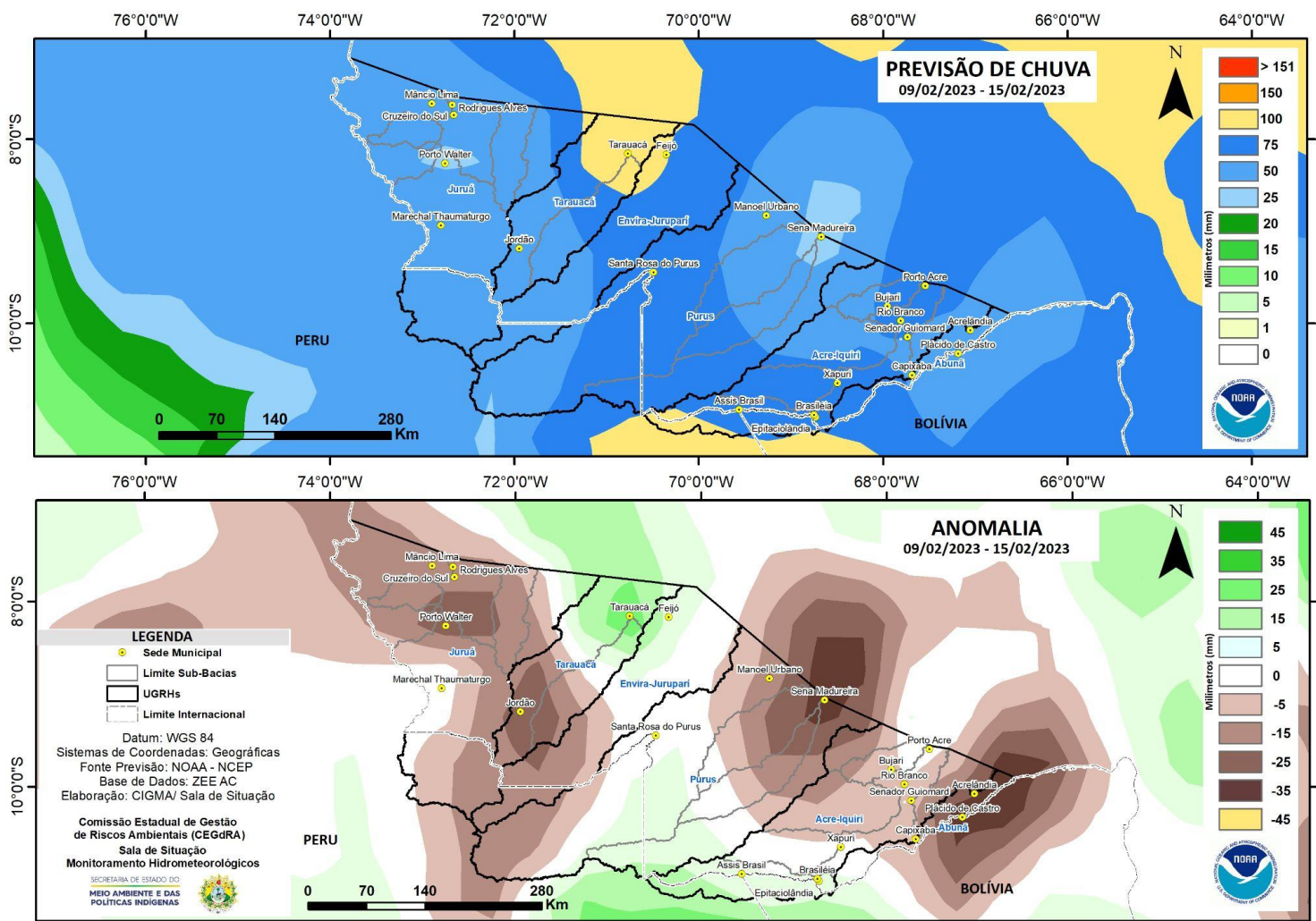
Figura 2: Prognóstico NCEP-GFS/USA.
