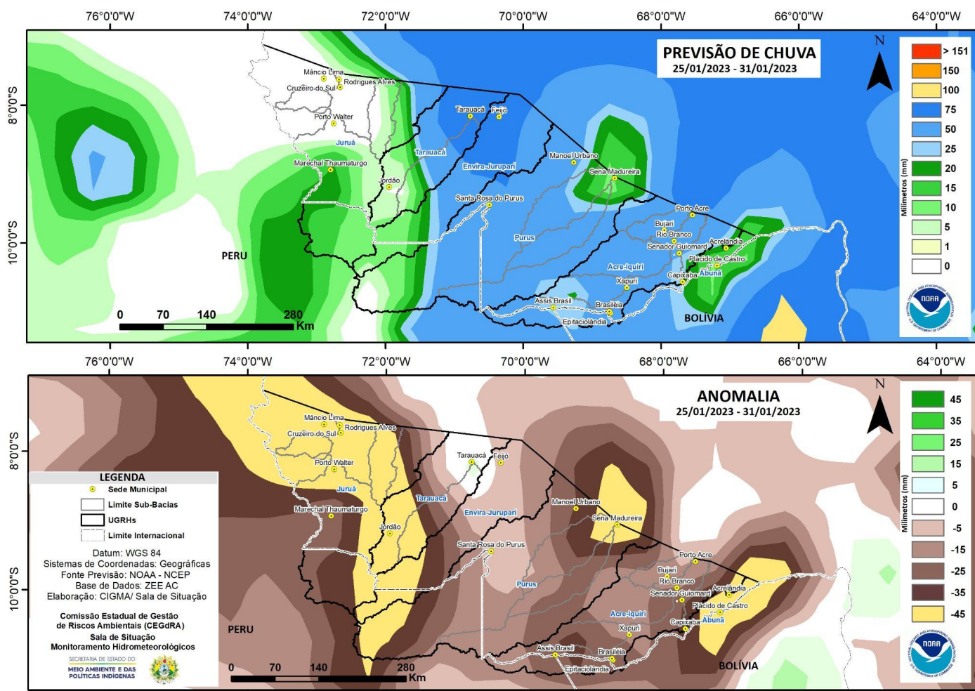
Figura 2: Prognóstico NCEP-GFS/USA.
