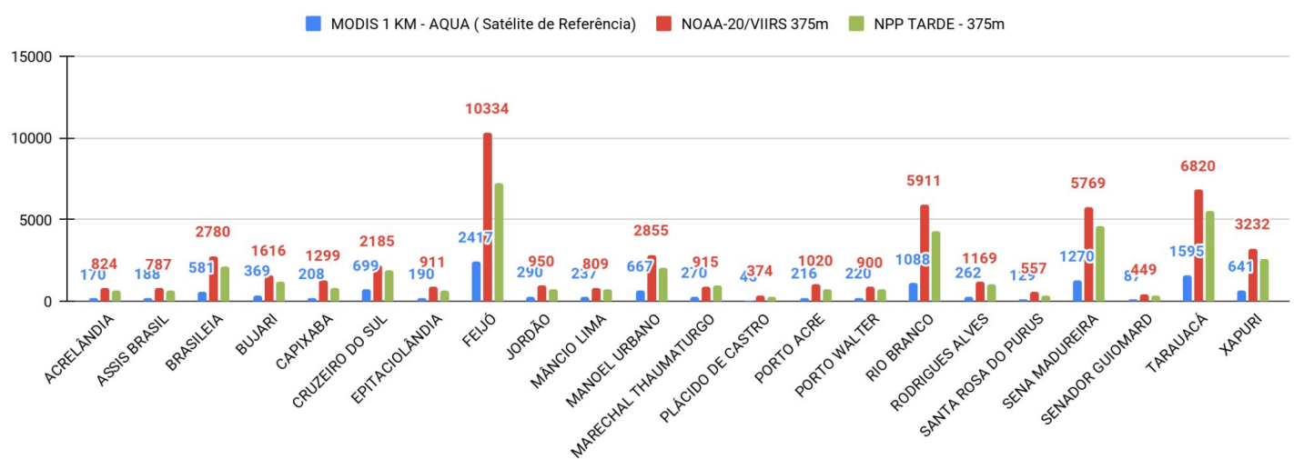
Figura 6 – Distribuição dos focos de queimadas acumulados de 01/01/2022 a 31/12/2022, no Estado do Acre. Satélite de referência AQUA (Barra de cor azul) e VIIRS 375m - NOAA-20 (Cor vermelha) e 375m - NPP TARDE (Cor verde)
