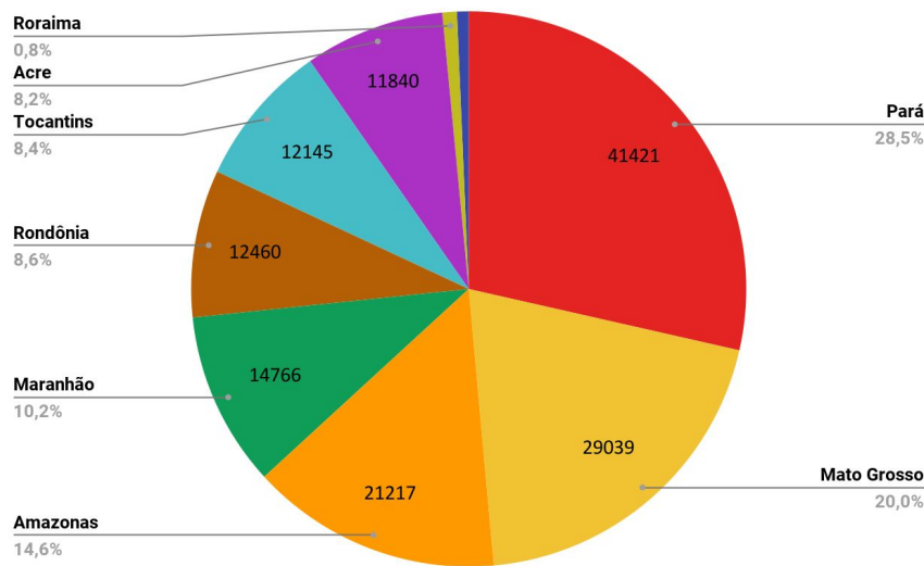
Figura 1 – Distribuição percentual dos focos de queimadas acumulados em 01/01/2022 a 31/12/2022 na Amazônia legal (Satélite de Referência AQUA)
