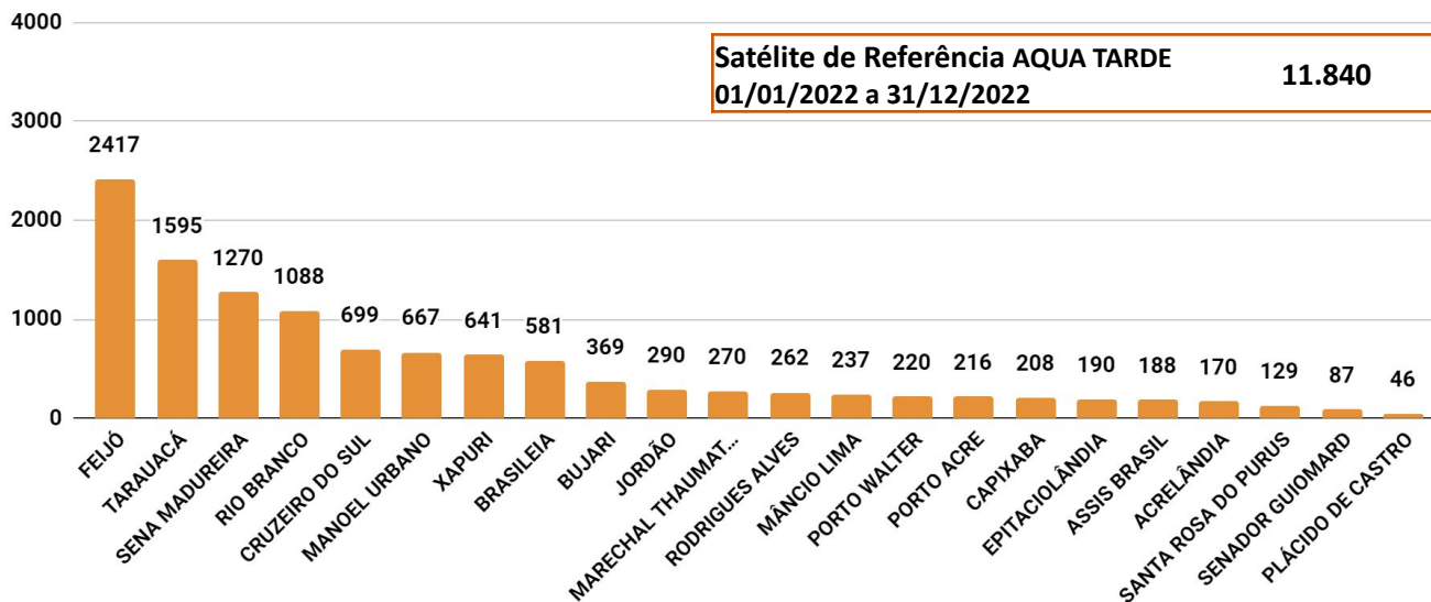
Figura 3 – Distribuição percentual dos focos de queimadas acumulados em 01/01/2022 a 31/12/2022 no estado do Acre (Satélite de Referência AQUA Tarde)
