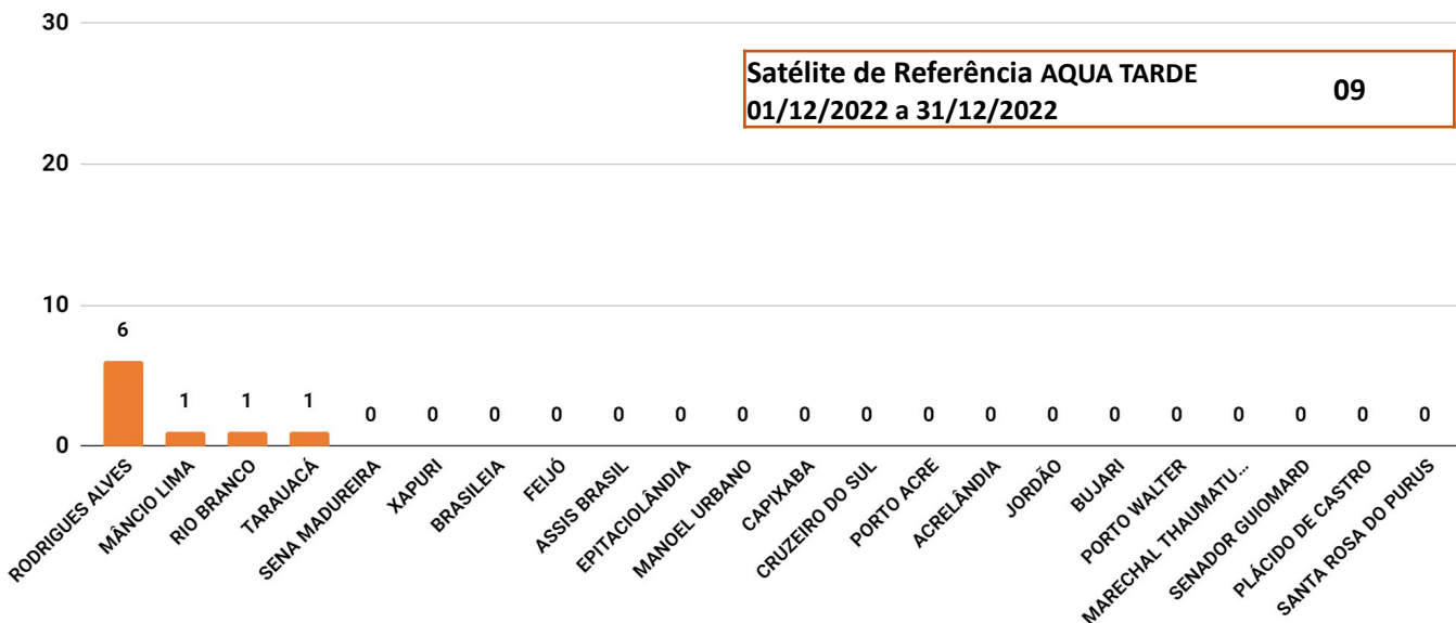
Figura 4 – Distribuição percentual dos focos de queimadas acumulados em 01/12/2022 a 31/12/2022 no estado do Acre (Satélite de Referência AQUA Tarde)
