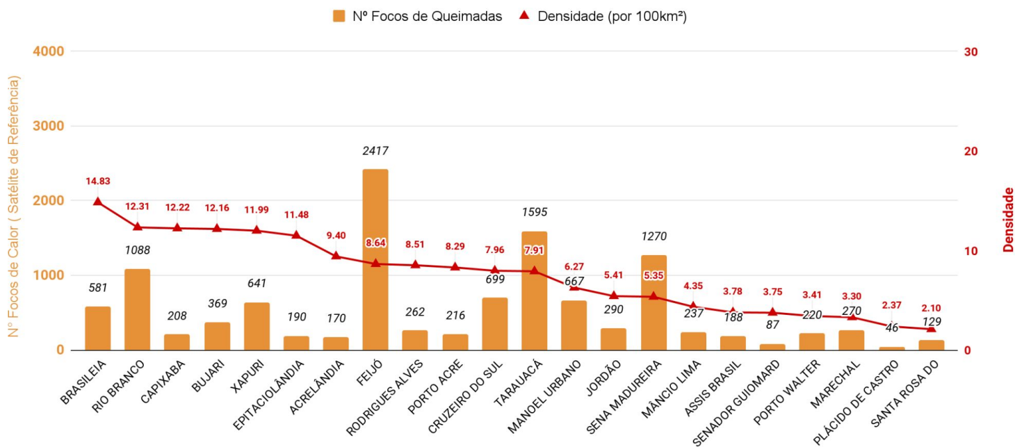
Figura 5 – Ocorrência de focos de queimadas e densidade por km 2 , por município em 01/01/2022 a 31/12/2022 (Satélite de referência AQUA)
