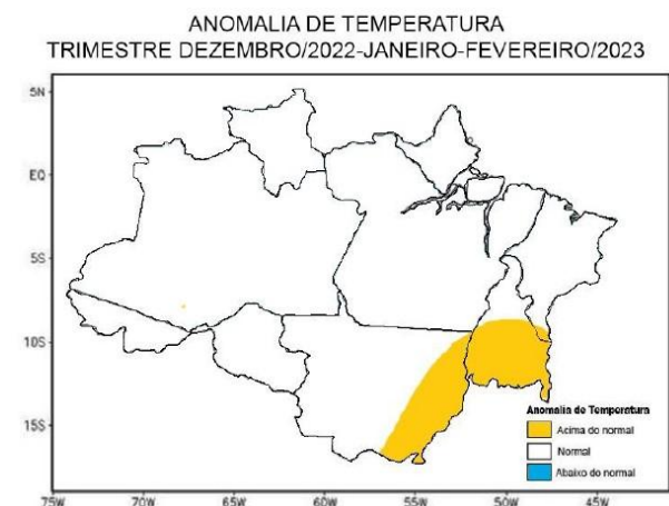
Figura 03 - Prognóstico de anomalias de temperatura para o trimestre Dezembro/2022 - Janeiro-Fevereiro/2023.
