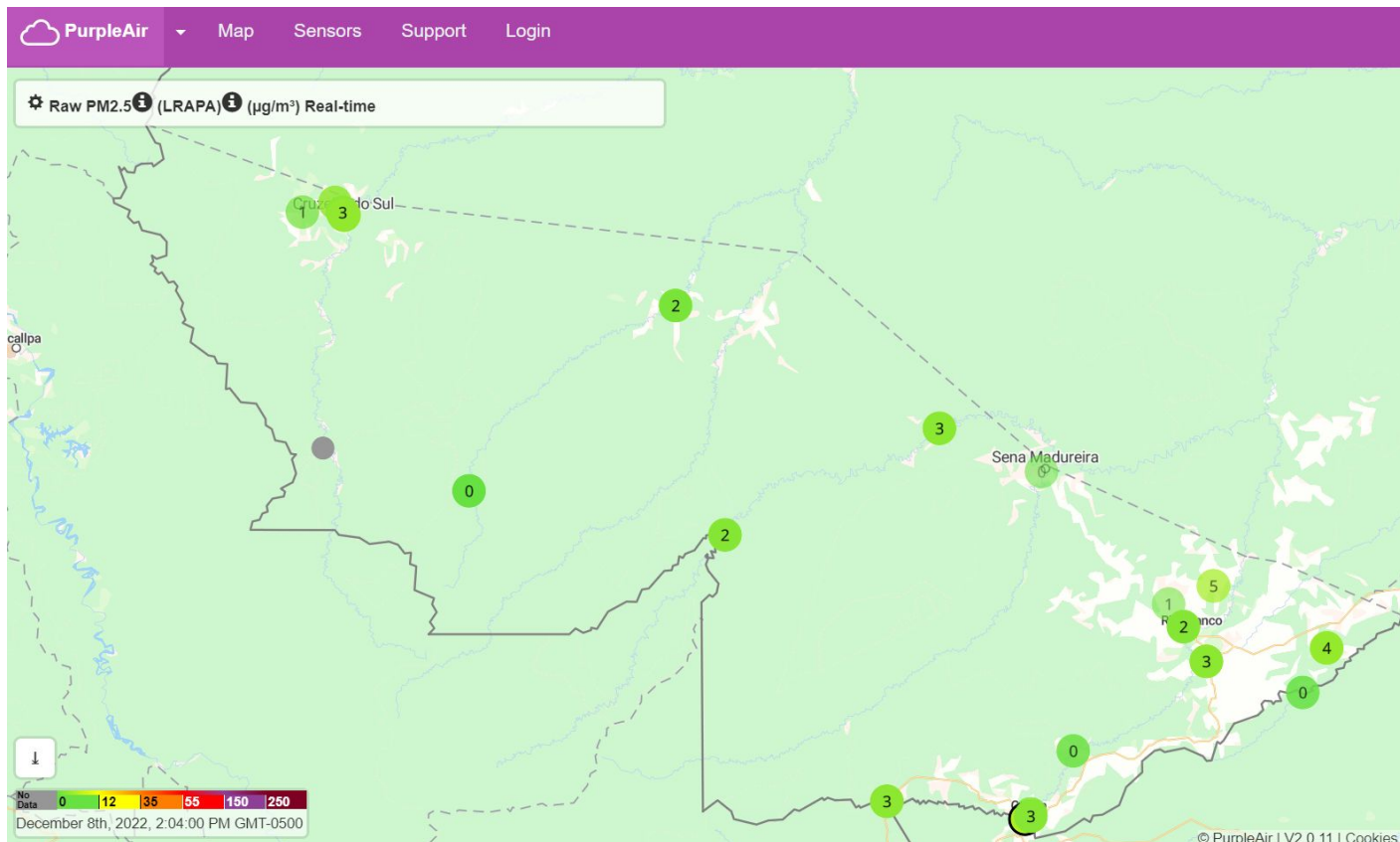
Figura 7 – Concentração de Material Particulado PM 2.5 \mu\text{g}/\text{m}^3 média para dia 08/12/2022 Dados coletados às 14h:04min
