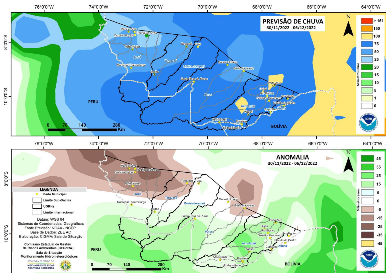
Figura 2: Prognóstico NCEP-GFS/USA.
