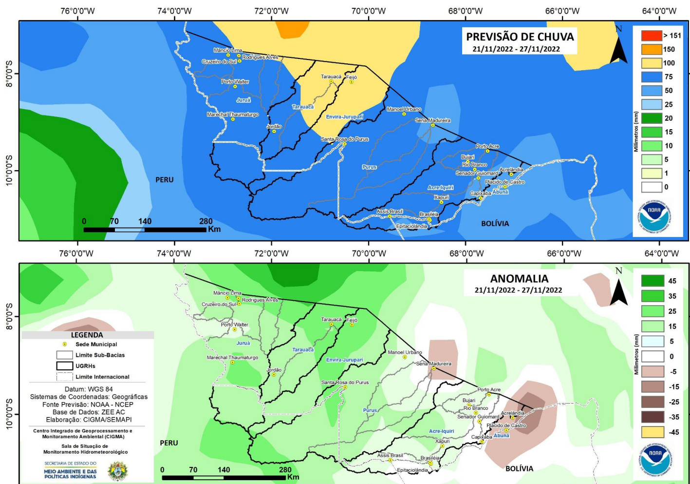
Figura 2: Prognóstico NCEP-GFS/USA.
