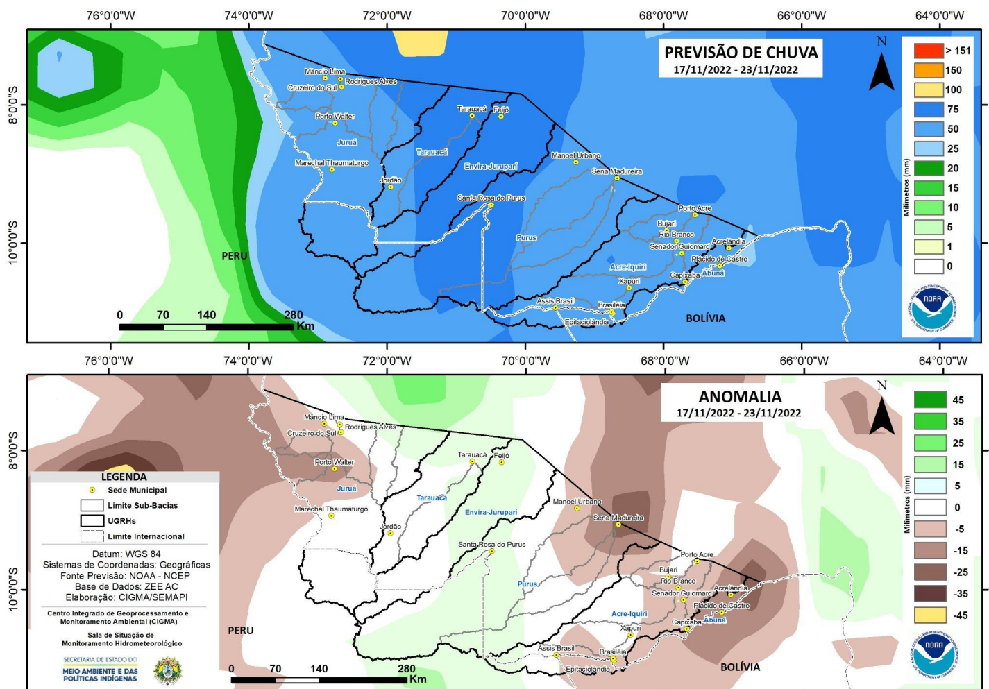
Figura 2: Prognóstico NCEP-GFS/USA.
