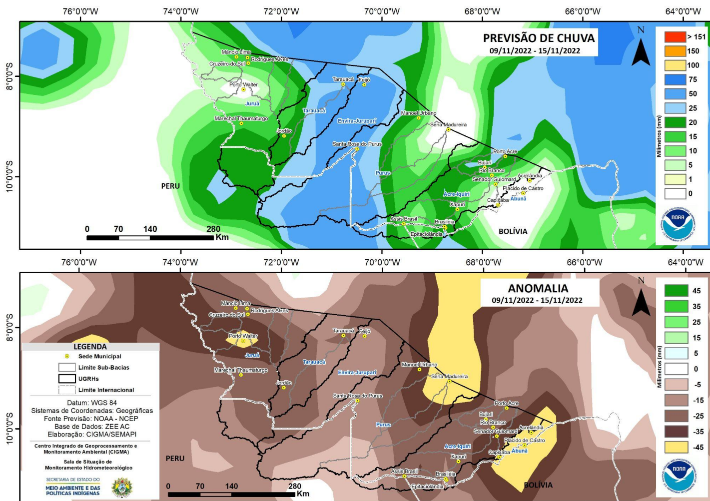
Figura 2: Prognóstico NCEP-GFS/USA.
