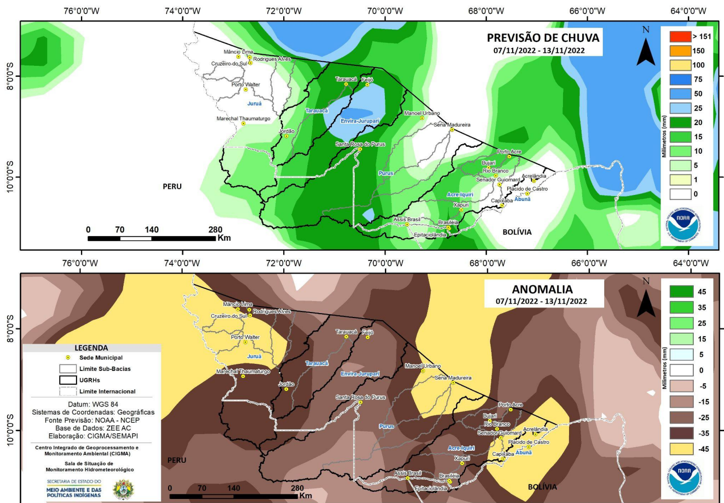
Figura 2: Prognóstico NCEP-GFS/USA.
