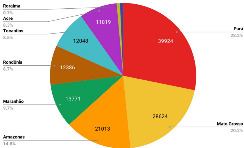
Figura 1 – Distribuição percentual dos focos de queimadas acumulados em 01/01/2022 a 29/11/2022 na Amazônia legal (Satélite de Referência AQUA)
