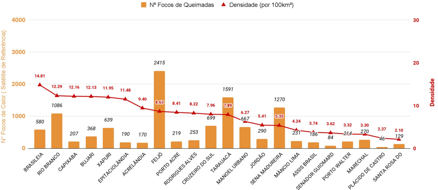
Figura 5 – Ocorrência de focos de queimadas e densidade por km 2 , por município em 01/01/2022 a 15/11/2022 (Satélite de referência AQUA)
