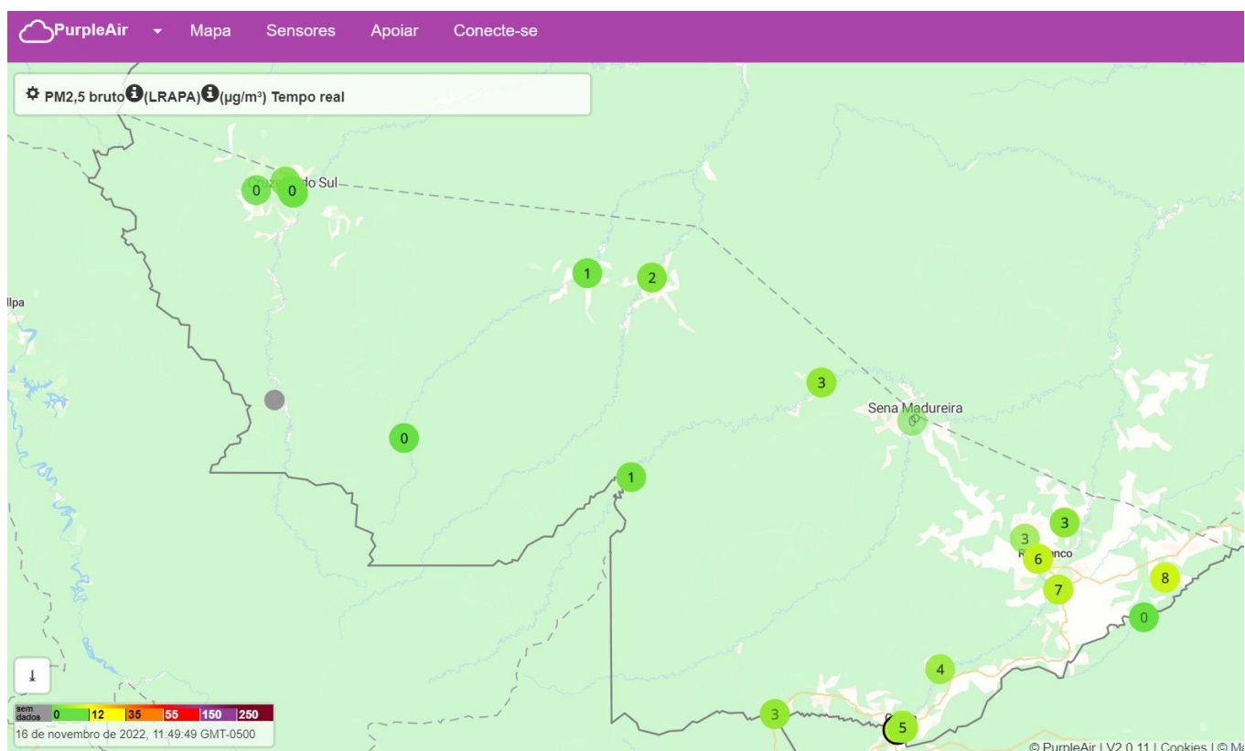
Figura 7 – Concentração de Material Particulado PM 2.5 \mu\text{g}/\text{m}^3 média para dia 16/11/2022 Dados coletados às 11h:50min
