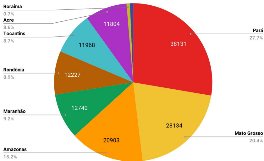
Figura 1 – Distribuição percentual dos focos de queimadas acumulados em 01/01/2022 a 15/11/2022 na Amazônia legal (Satélite de Referência AQUA)
