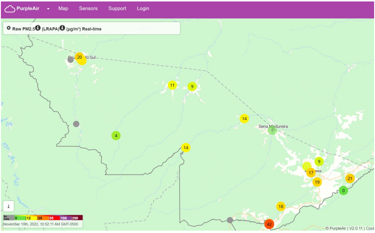
Figura 8 – Concentração de Material Particulado PM 2.5 \mu\text{g}/\text{m}^3 média para dia 10/11/2022 Dados coletados às 10h:52min
