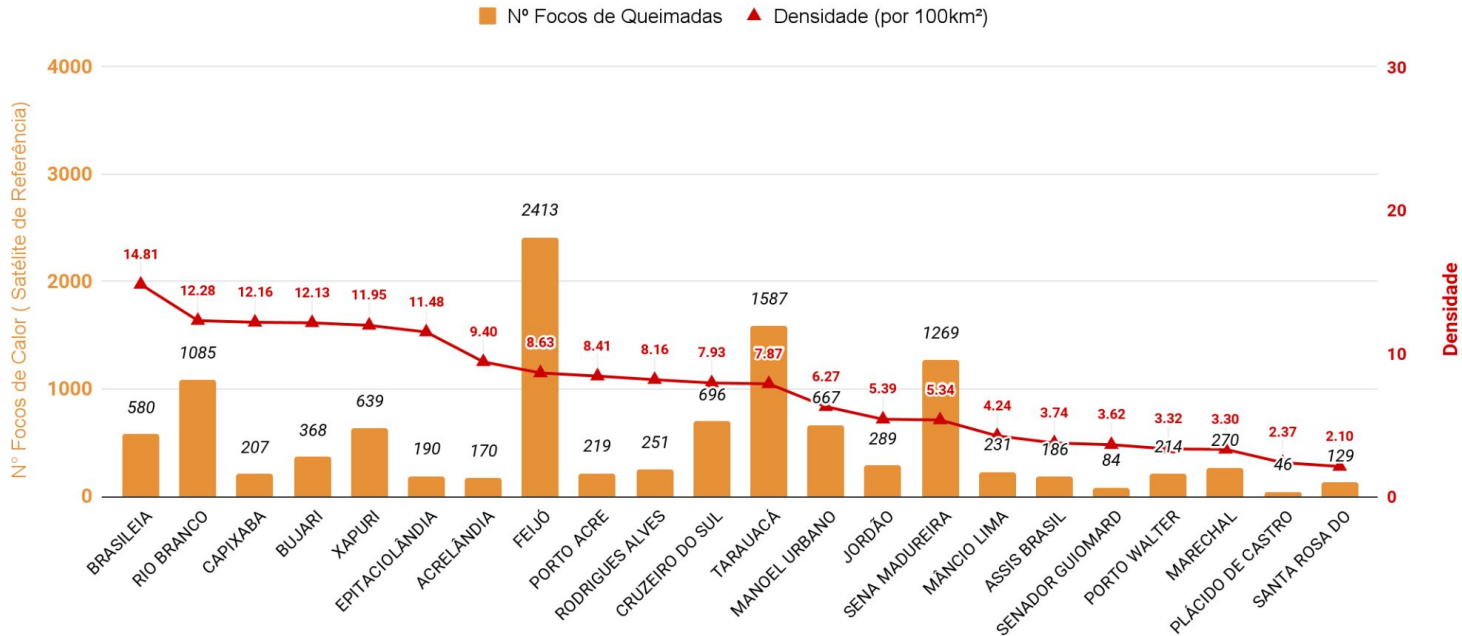
Figura 5 – Ocorrência de focos de queimadas e densidade por km 2 , por município em 01/01/2022 a 09/11/2022 (Satélite de referência AQUA)
