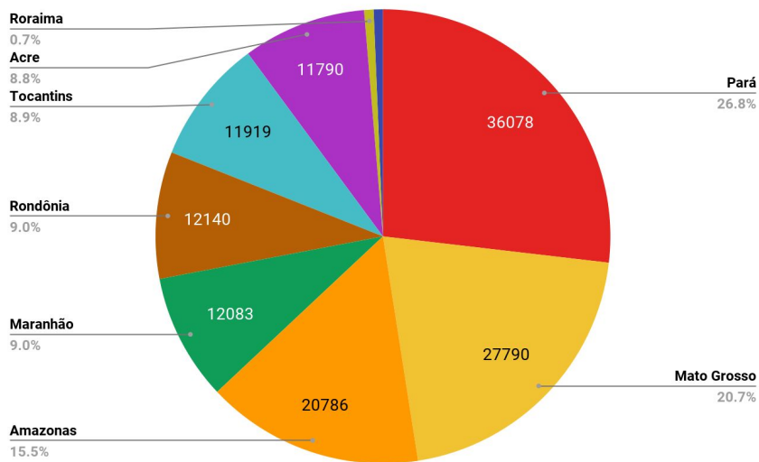
Figura 1 – Distribuição percentual dos focos de queimadas acumulados em 01/01/2022 a 09/11/2022 na Amazônia legal (Satélite de Referência AQUA)
