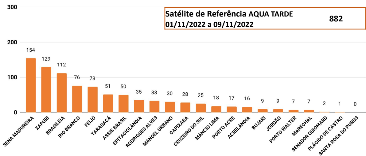
Figura 4 – Distribuição percentual dos focos de queimadas acumulados em 01/11/2022 a 09/11/2022 no estado do Acre (Satélite de Referência AQUA Tarde)
