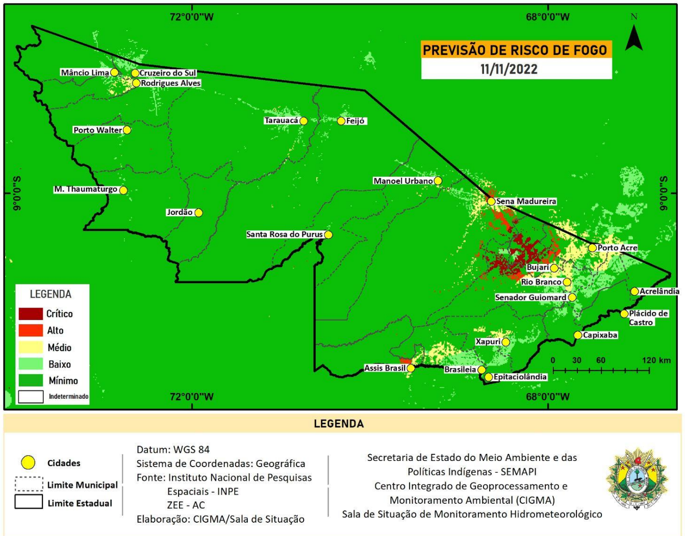
Figura 7 – Risco de Fogo previsto para o estado do Acre para amanhã 11/11/2022
