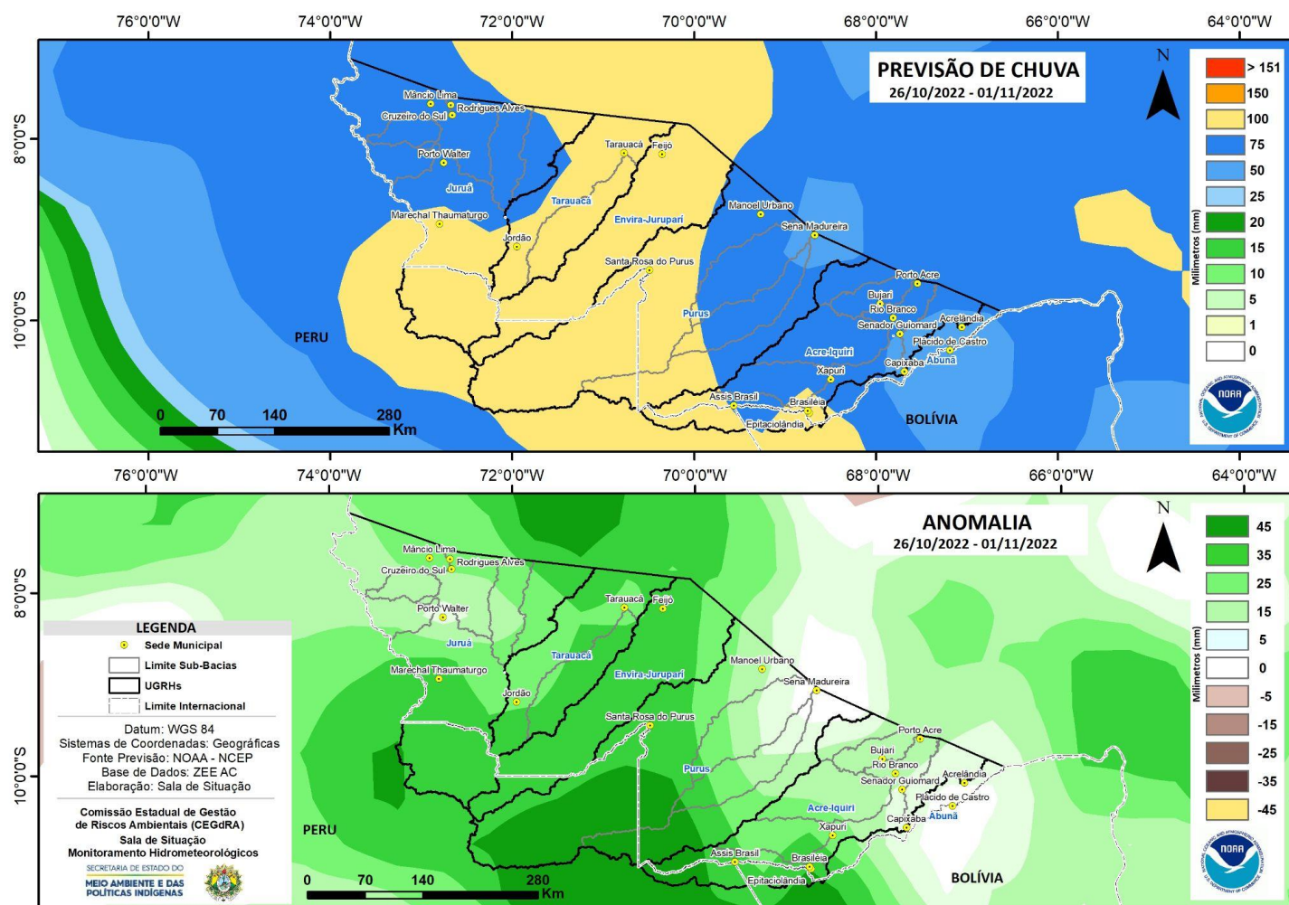
Figura 2: Prognóstico NCEP-GFS/USA.
