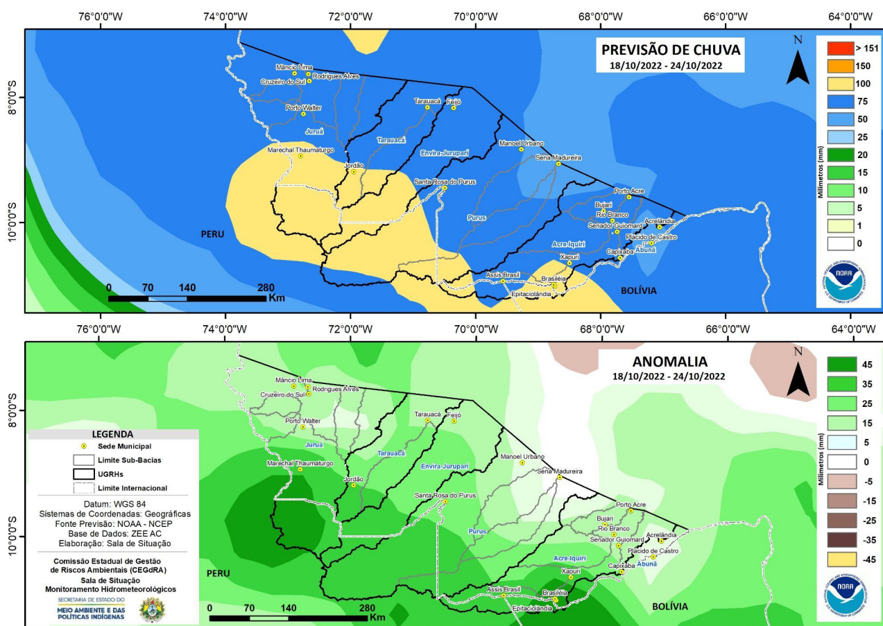
Figura 2: Prognóstico NCEP-GFS/USA.
