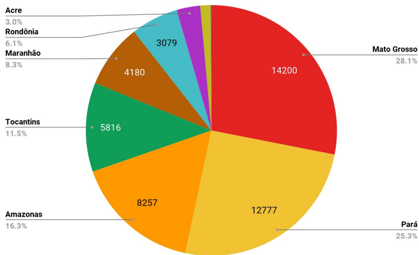
Figura 1 – Distribuição percentual dos focos de queimadas acumulados em 01/01/2022 a 24/08/2022 na Amazônia legal (Satélite de Referência AQUA)
