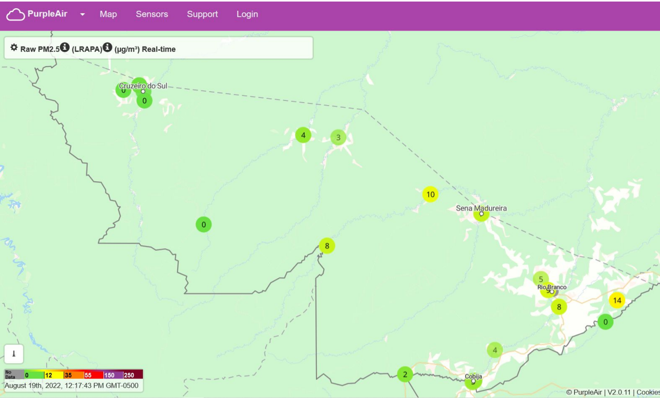
Figura 8 – Concentração de Material Particulado PM 2.5 \mu\text{g}/\text{m}^3 média para dia 19/08/2022.
