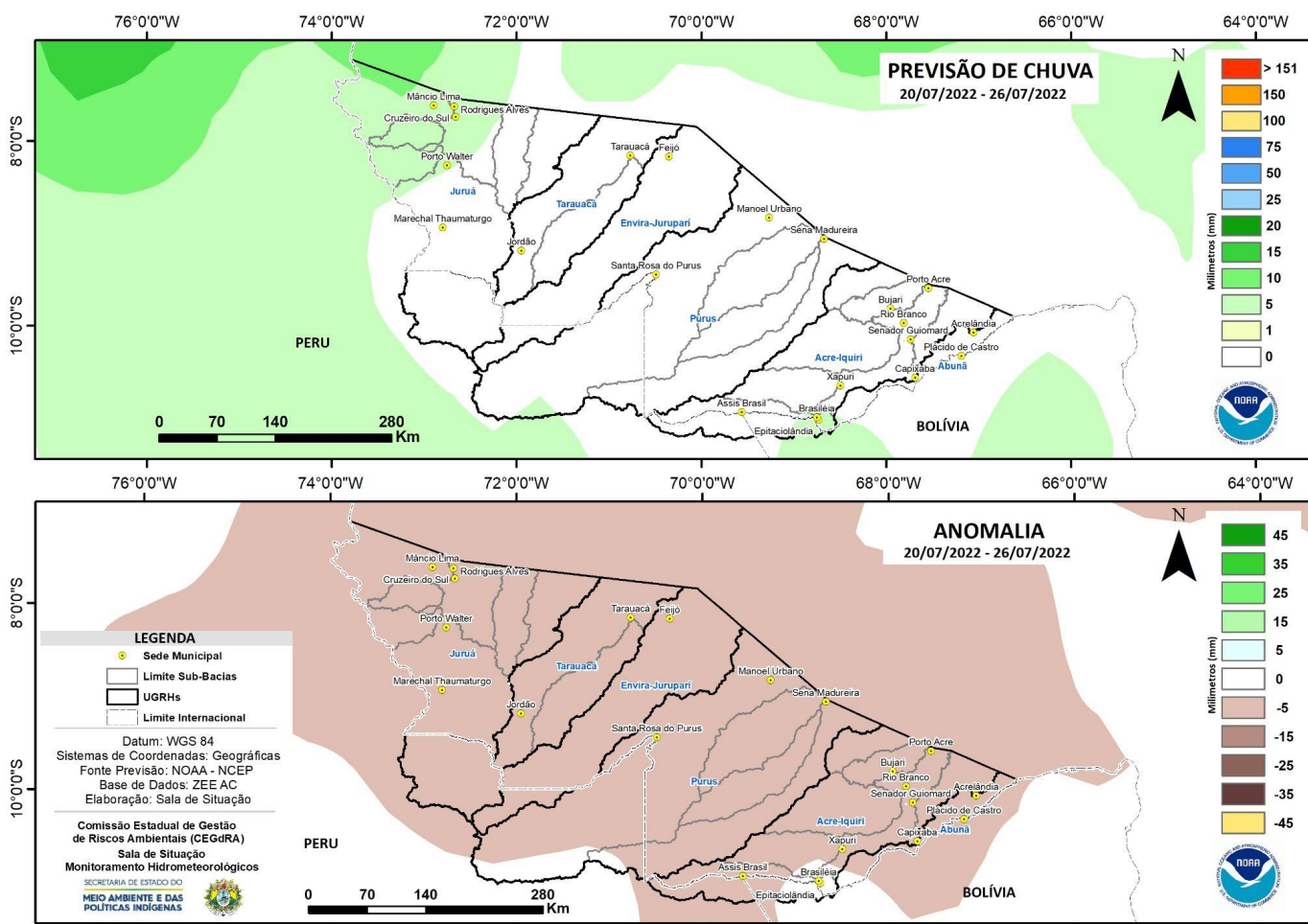
Figura 2: Prognóstico NCEP-GFS/USA.
