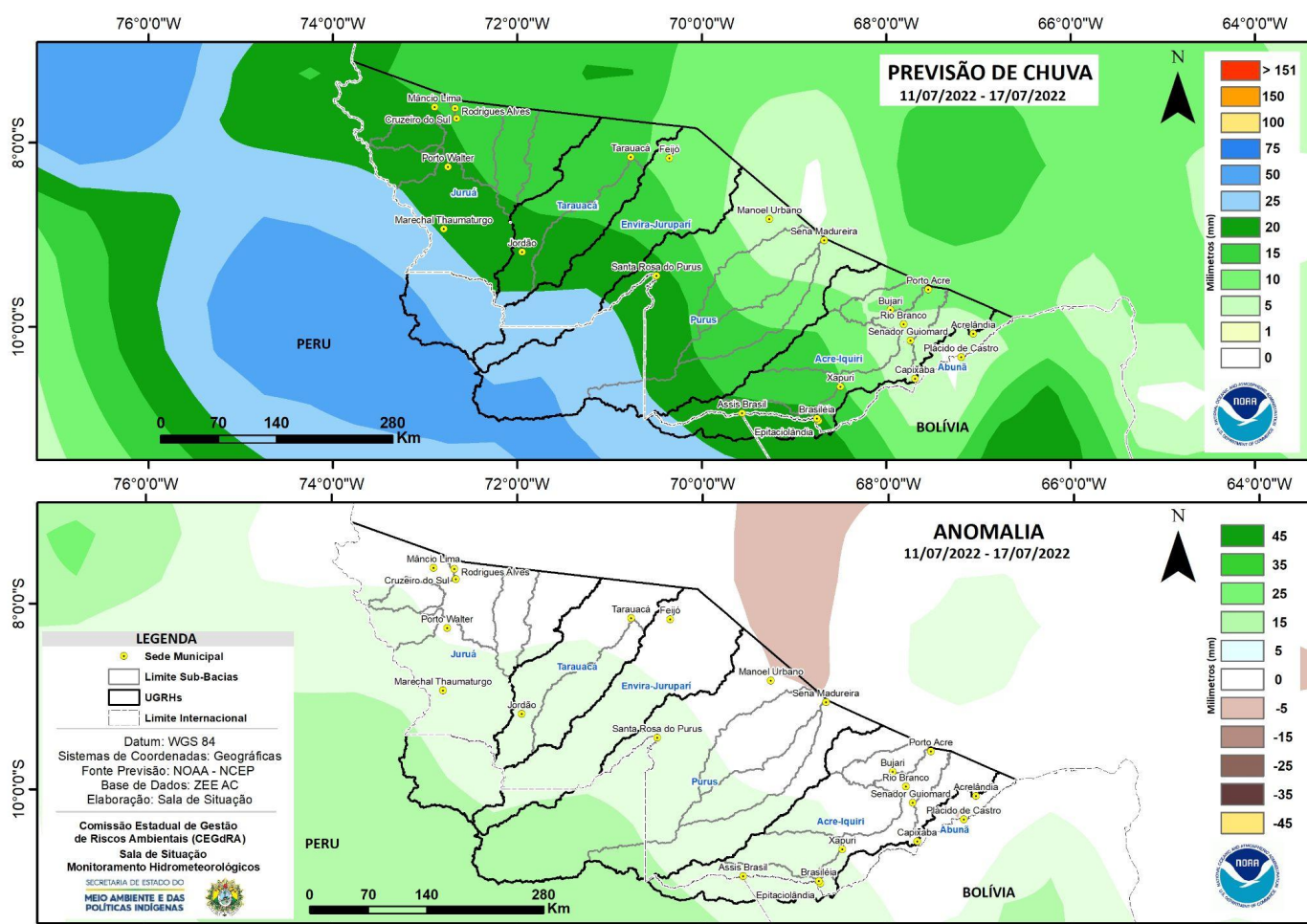
Figura 2: Prognóstico NCEP-GFS/USA.
