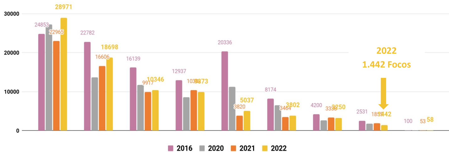
Figura 4 – Distribuição percentual dos focos de queimadas acumulados em 01/01/2022 a 27/07/2022 na Amazônia legal (Satélite S-NPP - 375 TARDE)
