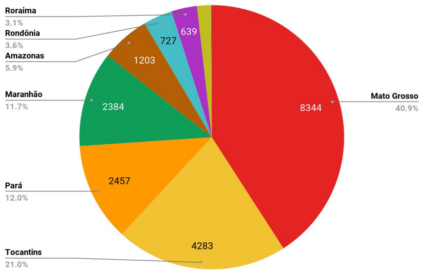
Figura 1 – Distribuição percentual dos focos de queimadas acumulados em 01/01/2022 a 27/07/2022 na Amazônia legal (Satélite de Referência AQUA)
