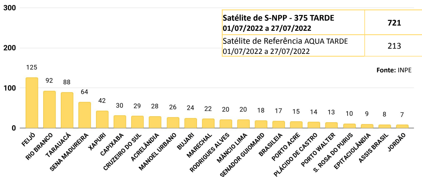
Figura 6 – Distribuição percentual dos focos de queimadas acumulados em 01/07/2022 a 27/07/2022 no estado do Acre (Satélite S-NPP - 375 TARDE)
