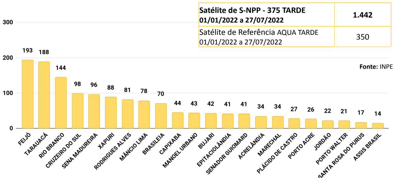
Figura 6 – Distribuição percentual dos focos de queimadas acumulados em 01/01/2022 a 27/07/2022 no estado do Acre (Satélite S-NPP - 375 TARDE)
