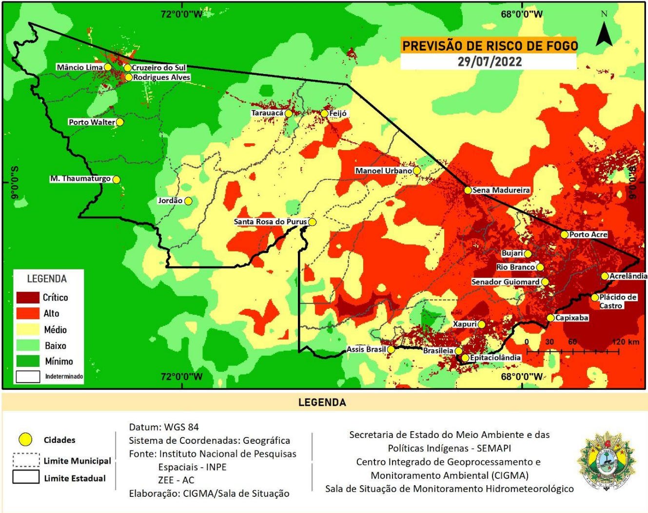
Figura 9 – Distribuição do Risco de Fogo previsto para o estado do Acre para amanhã 29/07/2022
