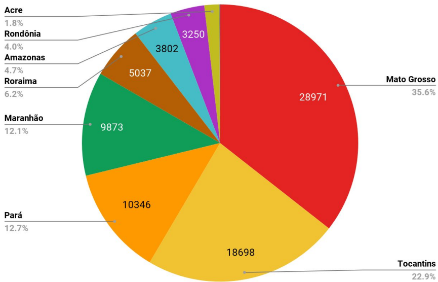
Figura 2 – Distribuição percentual dos focos de queimadas acumulados em 01/01/2022 a 27/07/2022 na Amazônia legal (Satélite S-NPP - 375 TARDE)
