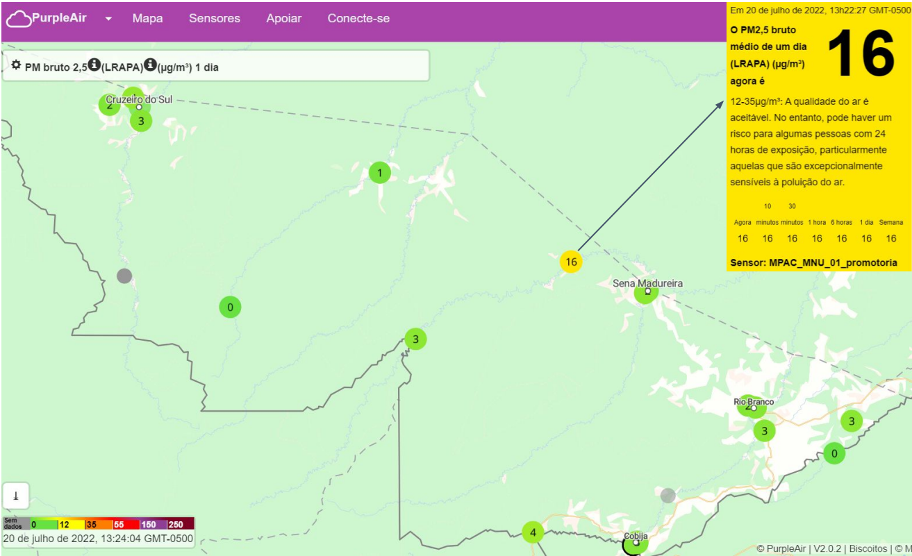
Figura 10 – Concentração de Material Particulado PM 2.5 \mu\text{g}/\text{m}^3 média para dia 20/07/2022.
