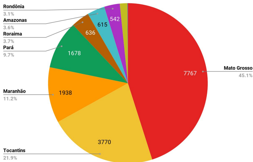
Figura 1 – Distribuição percentual dos focos de queimadas acumulados em 01/01/2022 a 18/07/2022 na Amazônia legal (Satélite de Referência AQUA)
