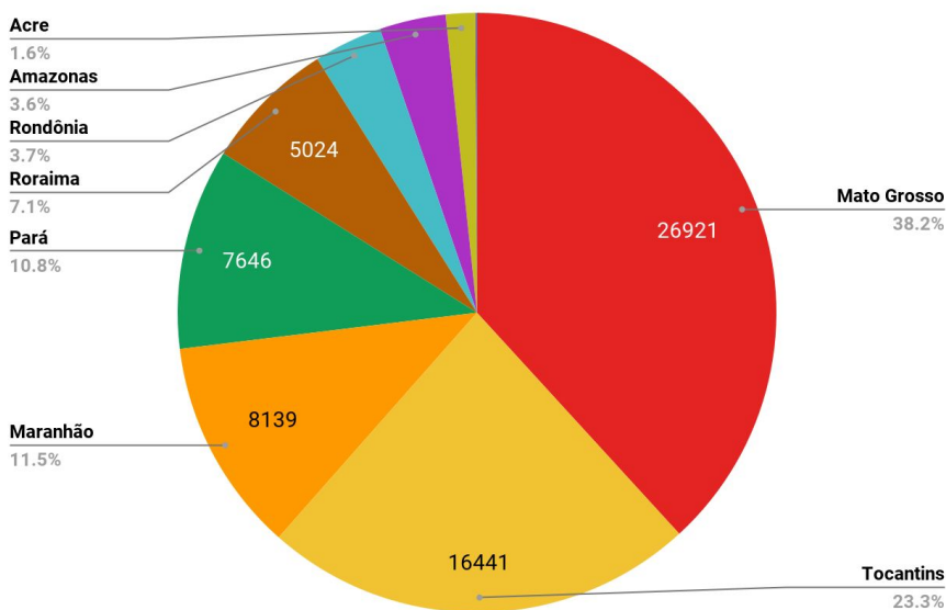
Figura 2 – Distribuição percentual dos focos de queimadas acumulados em 01/01/2022 a 18/07/2022 na Amazônia legal (Satélite S-NPP - 375 TARDE)
