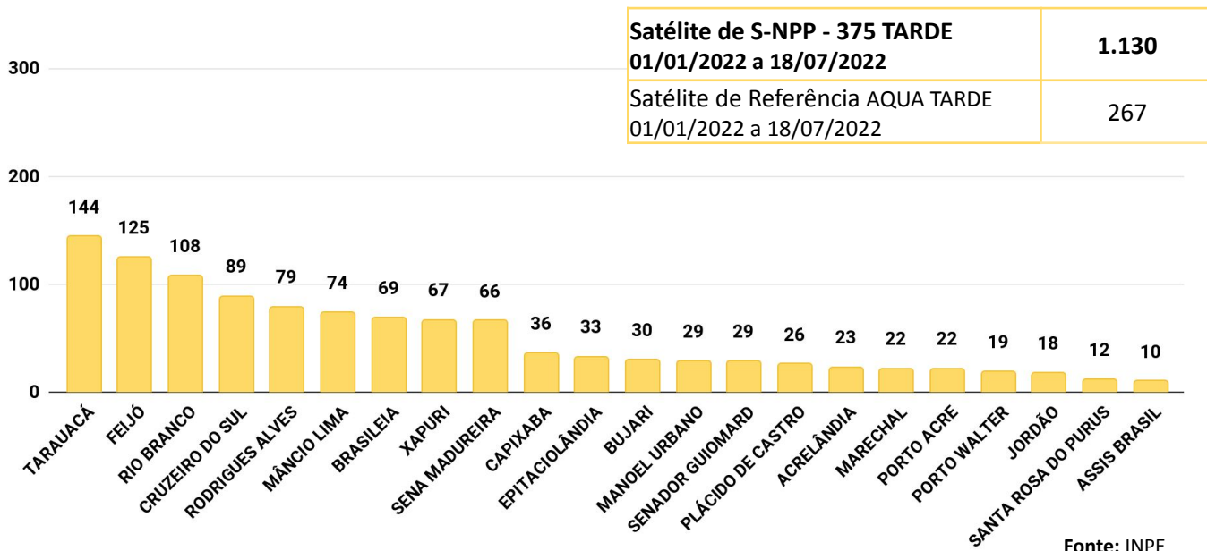
Figura 6 – Distribuição percentual dos focos de queimadas acumulados em 01/01/2022 a 18/07/2022 no estado do Acre (Satélite S-NPP - 375 TARDE)
