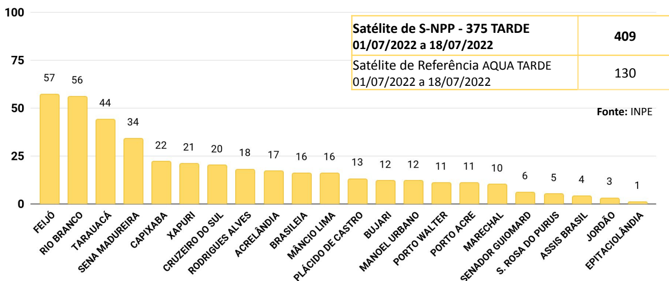
Figura 6 – Distribuição percentual dos focos de queimadas acumulados em 01/07/2022 a 18/07/2022 no estado do Acre (Satélite S-NPP - 375 TARDE)
