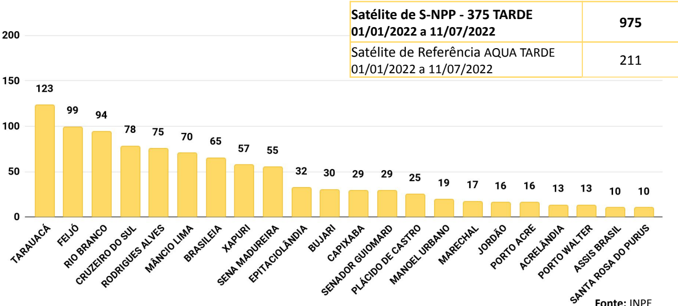
Figura 6 – Distribuição percentual dos focos de queimadas acumulados em 01/01/2022 a 11/07/2022 no estado do Acre (Satélite S-NPP - 375 TARDE)
