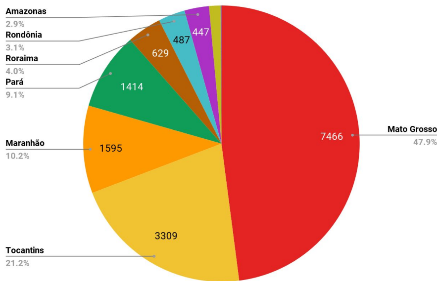
Figura 1 – Distribuição percentual dos focos de queimadas acumulados em 01/01/2022 a 11/07/2022 na Amazônia legal (Satélite de Referência AQUA)
