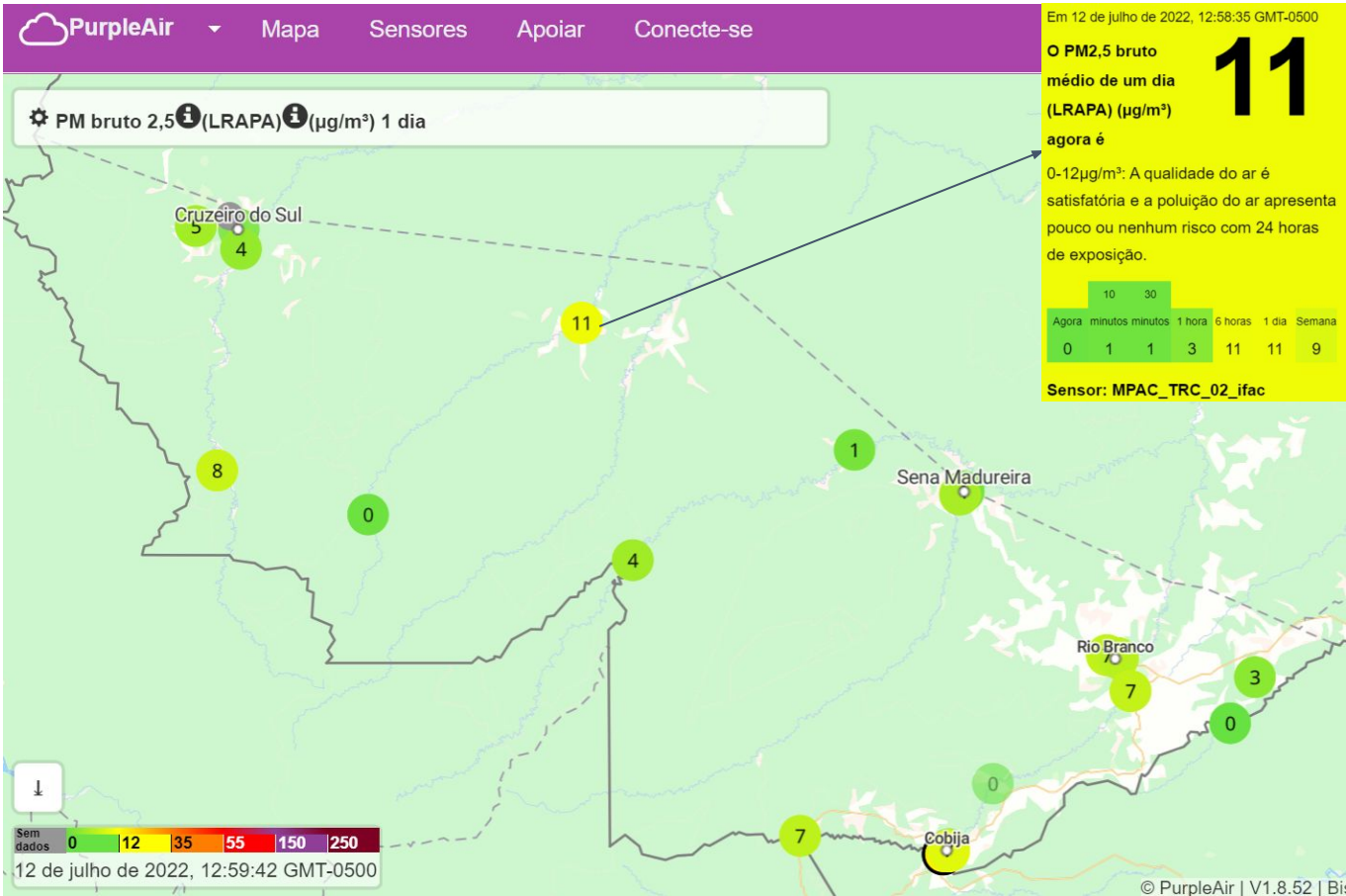
Figura 10 – Concentração de Material Particulado PM 2.5 \mu\text{g}/\text{m}^3 média para dia 12/07/2022.
