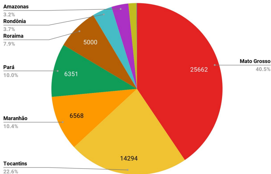
Figura 2 – Distribuição percentual dos focos de queimadas acumulados em 01/01/2022 a 11/07/2022 na Amazônia legal (Satélite S-NPP - 375 TARDE)
