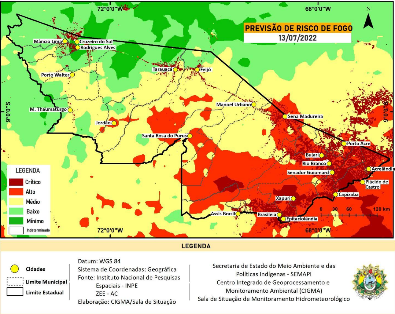
Figura 9 – Risco de Fogo previsto para o estado do Acre para amanhã 13/07/2022
