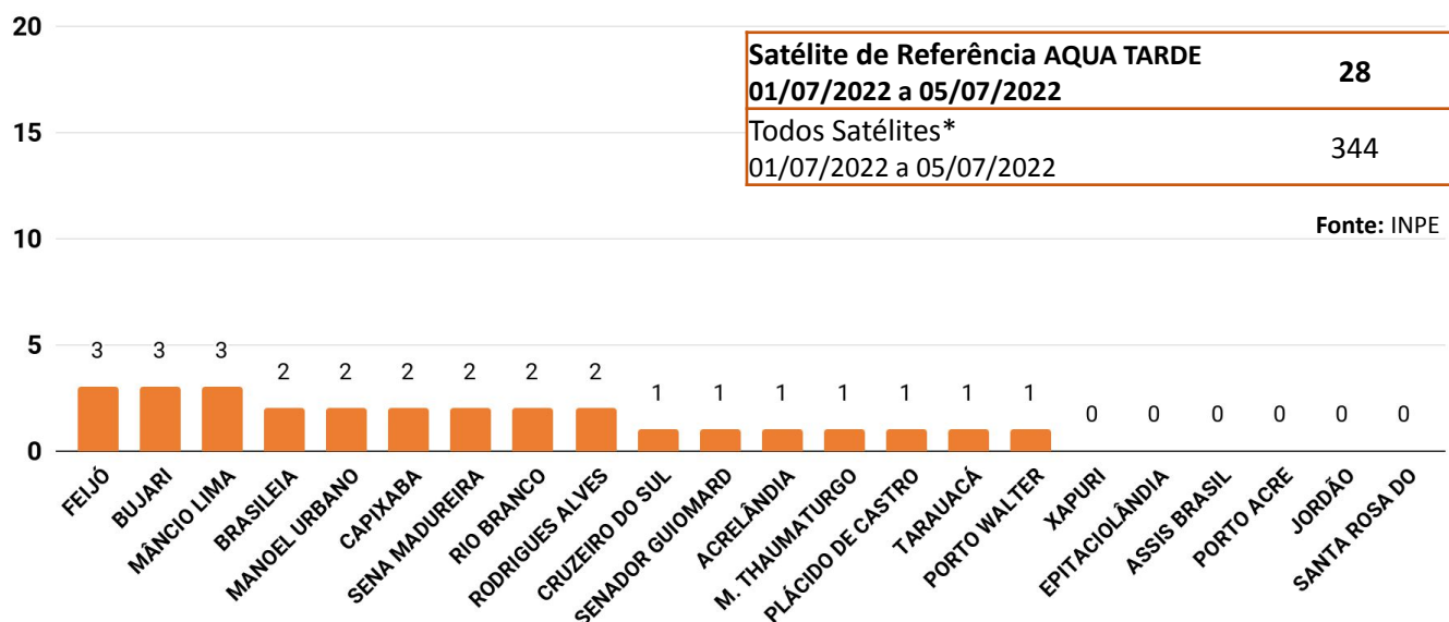
Figura 5 – Distribuição percentual dos focos de queimadas acumulados em 01/07/2022 a 05/07/2022 no estado do Acre (Satélite de Referência AQUA Tarde)
