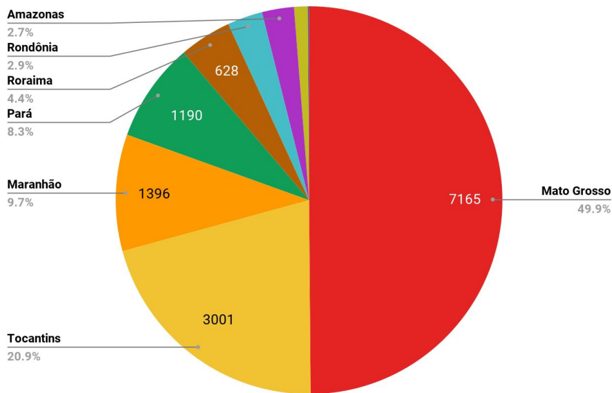
Figura 1 – Distribuição percentual dos focos de queimadas acumulados em 01/01/2022 a 05/07/2022 na Amazônia legal (Satélite de Referência AQUA)
