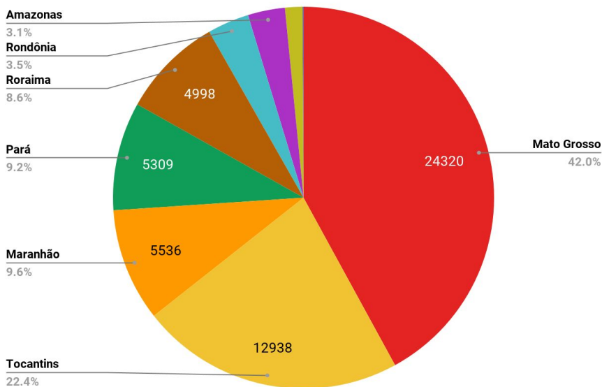
Figura 2 – Distribuição percentual dos focos de queimadas acumulados em 01/01/2022 a 05/07/2022 na Amazônia legal (Satélite S-NPP - 375 TARDE )
