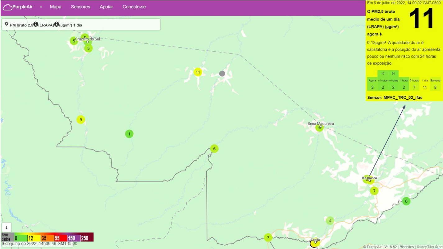
Figura 10 – Concentração de Material Particulado PM 2.5 \mu\text{g}/\text{m}^3 média para dia 06/07/2022.
