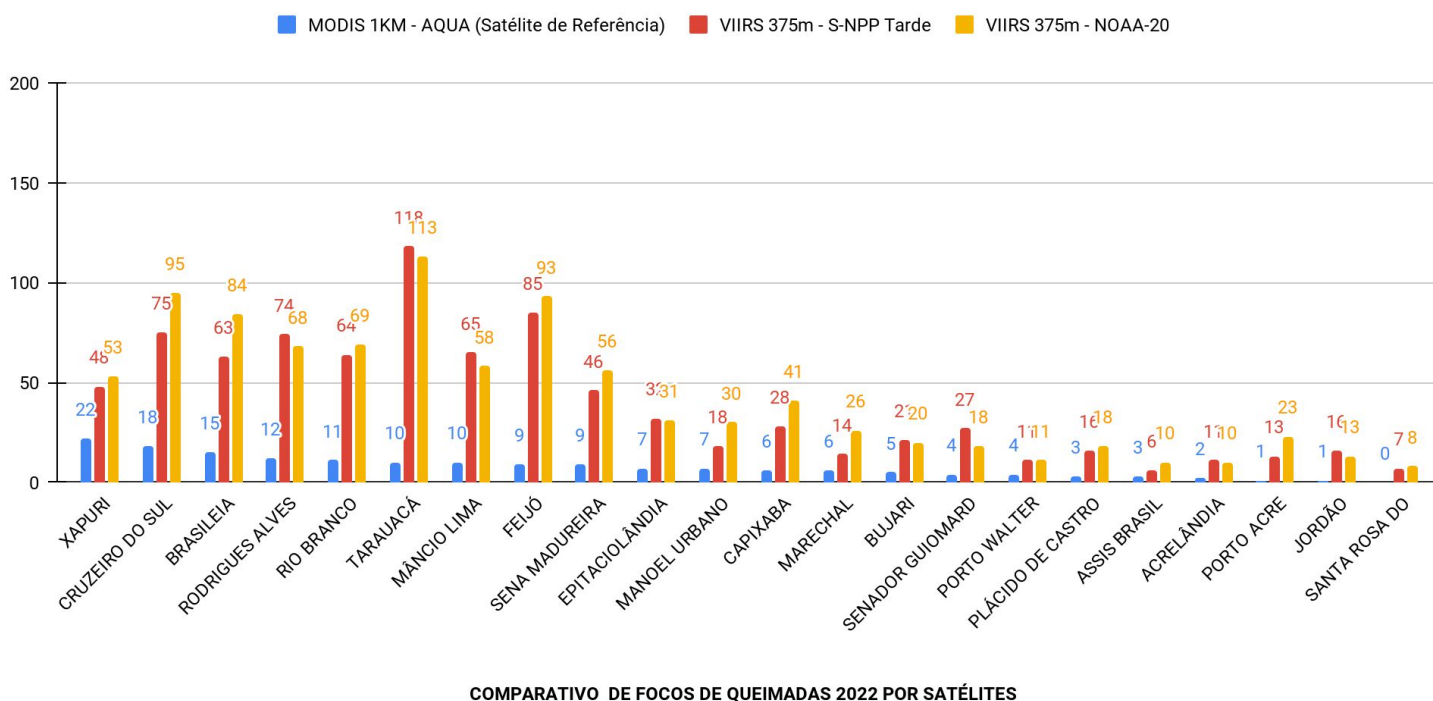
Figura 8 – Distribuição dos focos de queimadas acumulados de 01/01/2022 a 05/07/2022, no Estado do Acre. Satélite de referência AQUA (Barra de cor azul), VIIRS 375m/S-NPP Tarde (Cor vermelha) e VIIRS 375m - NOAA-20 (Cor amarela)
