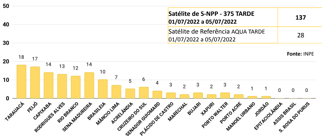
Figura 6 – Distribuição percentual dos focos de queimadas acumulados em 01/07/2022 a 05/07/2022 no estado do Acre (Satélite S-NPP - 375 TARDE)
