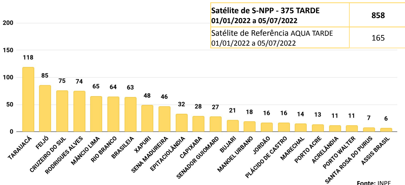
Figura 6 – Distribuição percentual dos focos de queimadas acumulados em 01/01/2022 a 05/07/2022 no estado do Acre (Satélite S-NPP - 375 TARDE)
