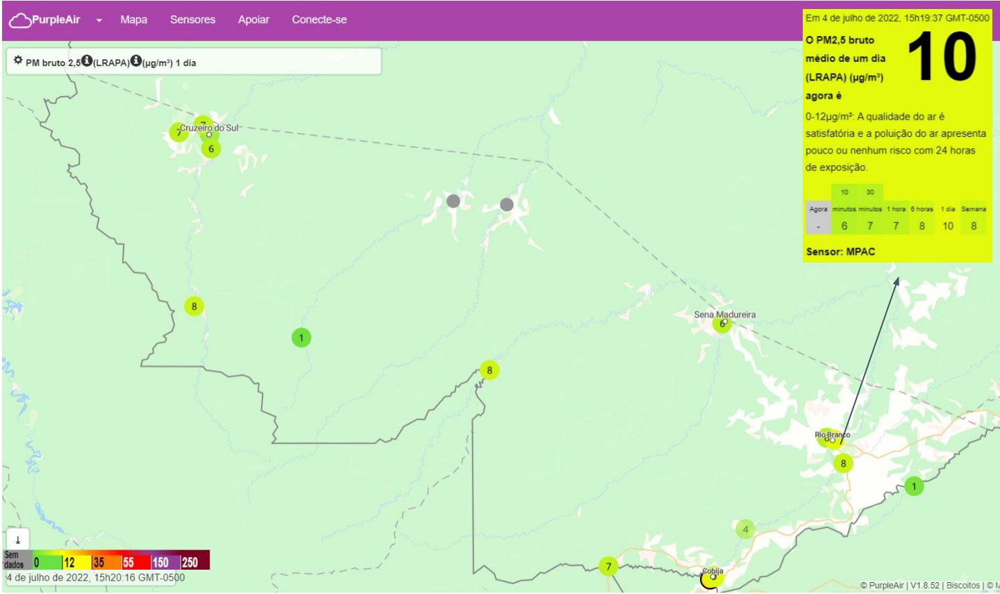
Figura 9 – Concentração de Material Particulado PM 2.5 \mu\text{g}/\text{m}^3 média para dia 04/07/2022.
