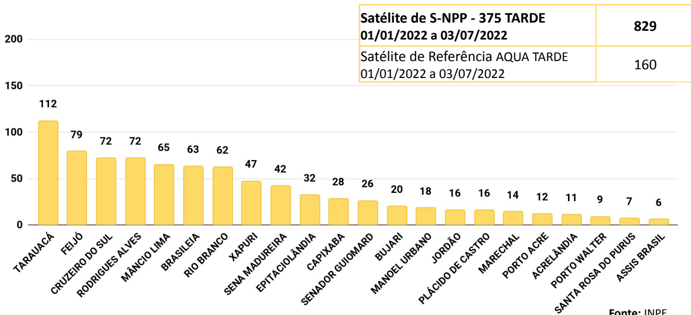
Figura 6 – Distribuição percentual dos focos de queimadas acumulados em 01/01/2022 a 03/07/2022 no estado do Acre (Satélite S-NPP - 375 TARDE)
