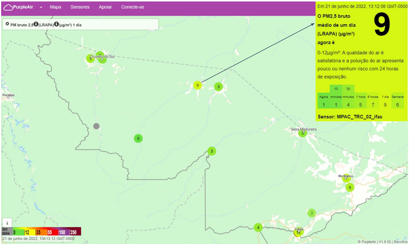
Figura 10 – Concentração de Material Particulado PM 2.5 \mu\text{g}/\text{m}^3 média para dia 21/06/2022.
