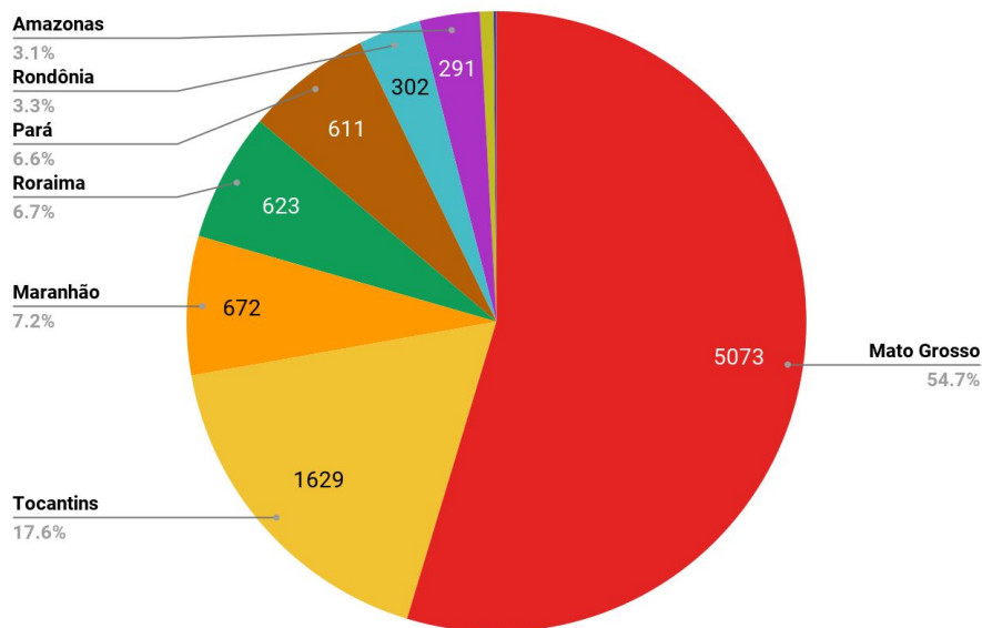
Figura 1 – Distribuição percentual dos focos de queimadas acumulados em 01/01/2022 a 07/06/2022 na Amazônia legal (Satélite de Referência AQUA)
