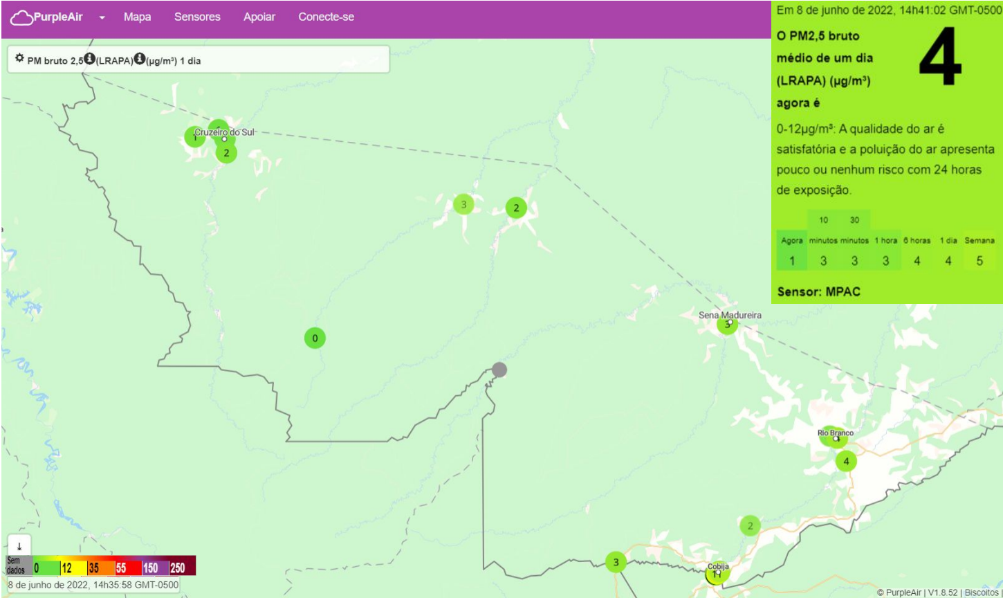
Figura 10 – Concentração de Material Particulado PM 2.5 \mu\text{g}/\text{m}^3 média para dia 08/06/2022.
