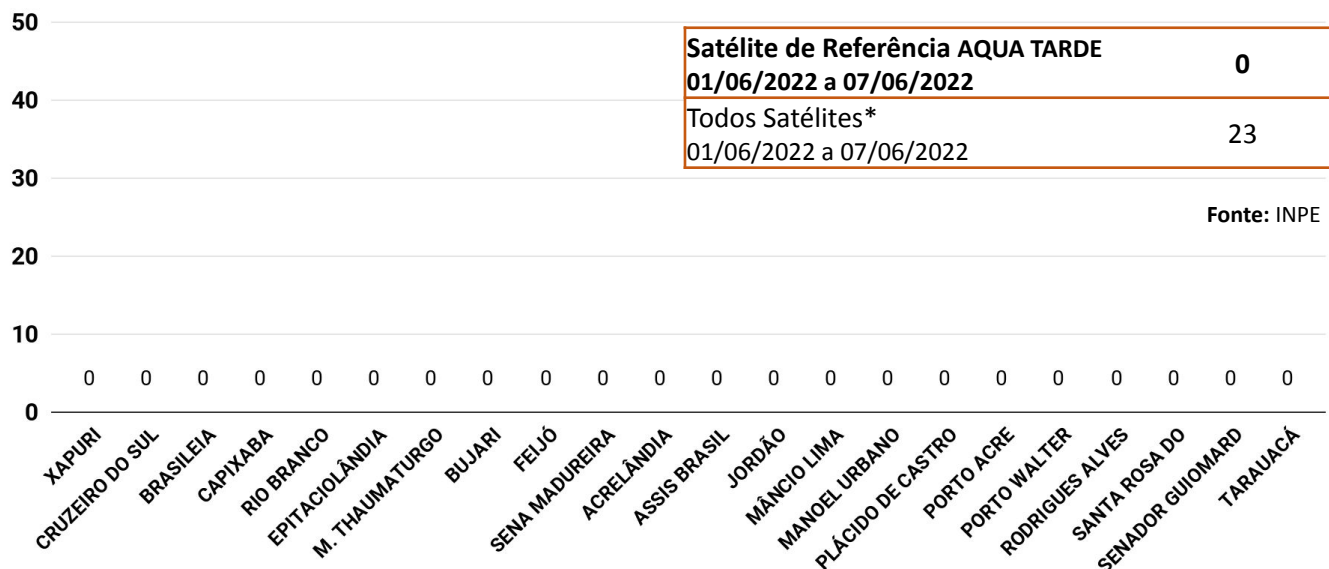
Figura 5 – Distribuição percentual dos focos de queimadas acumulados em 01/06/2022 a 07/06/2022 no estado do Acre (Satélite de Referência AQUA Tarde)
