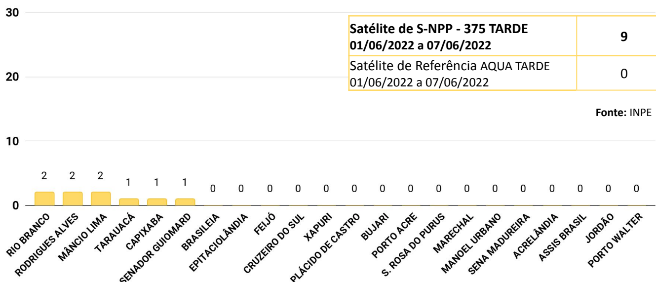
Figura 6 – Distribuição percentual dos focos de queimadas acumulados em 01/06/2022 a 07/06/2022 no estado do Acre (Satélite S-NPP - 375 TARDE)
