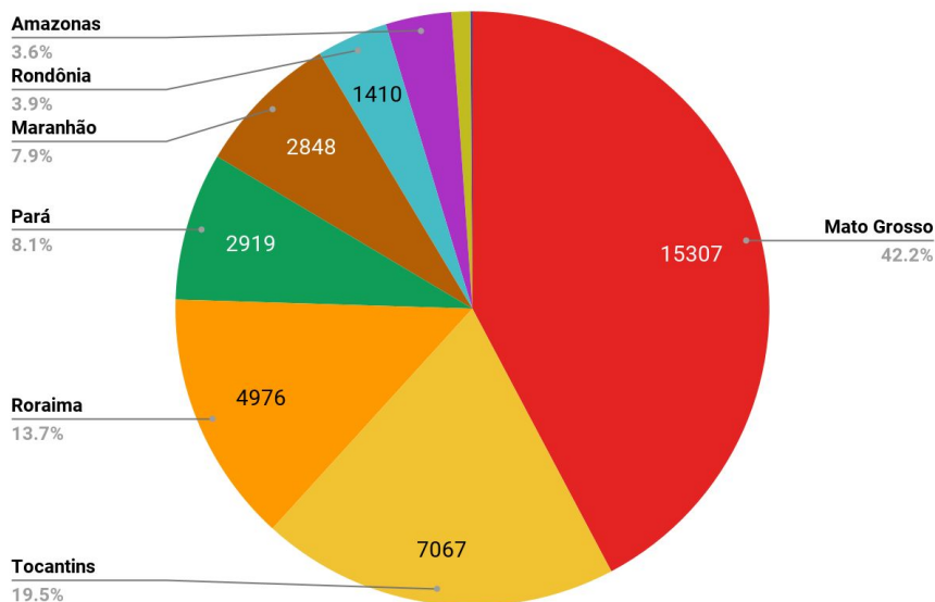
Figura 2 – Distribuição percentual dos focos de queimadas acumulados em 01/01/2022 a 07/06/2022 na Amazônia legal (Satélite S-NPP - 375 TARDE)
