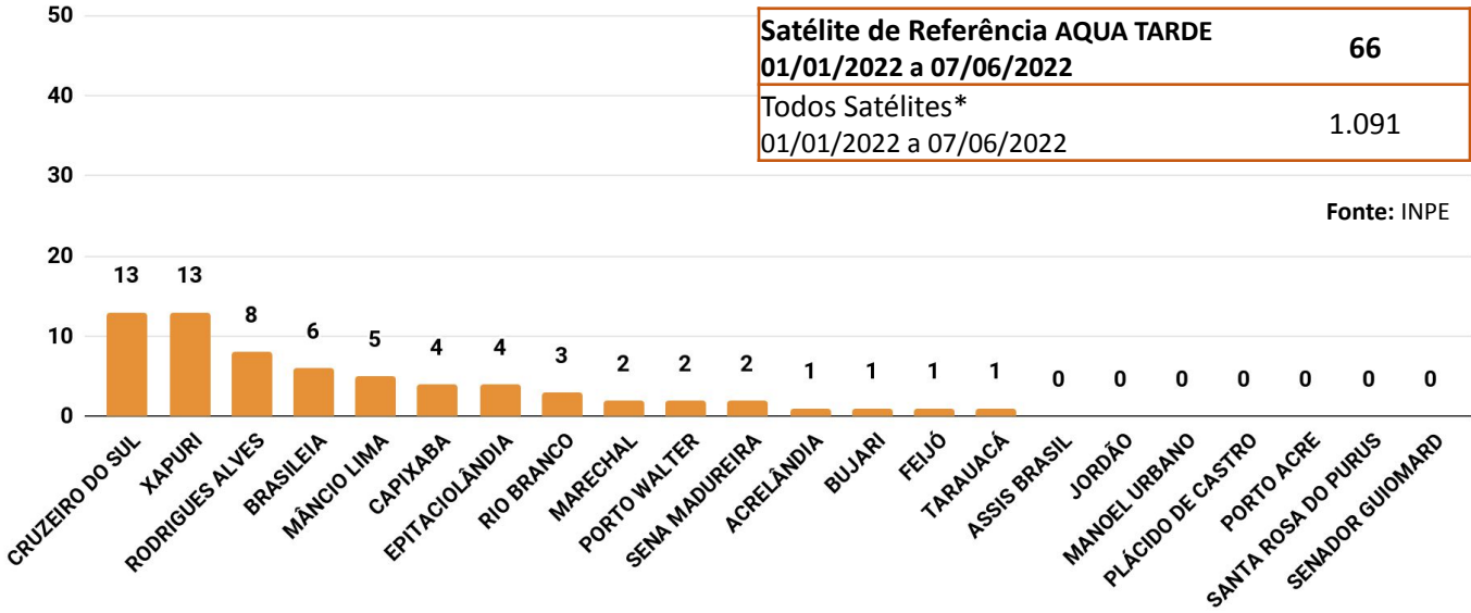
Figura 5 – Distribuição percentual dos focos de queimadas acumulados em 01/01/2022 a 07/06/2022 no estado do Acre (Satélite de Referência AQUA Tarde)
