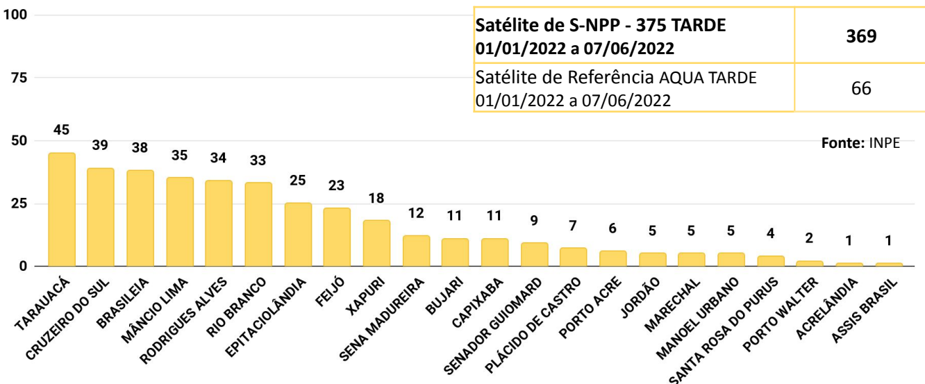
Figura 6 – Distribuição percentual dos focos de queimadas acumulados em 01/01/2022 a 07/06/2022 no estado do Acre (Satélite S-NPP - 375 TARDE)
