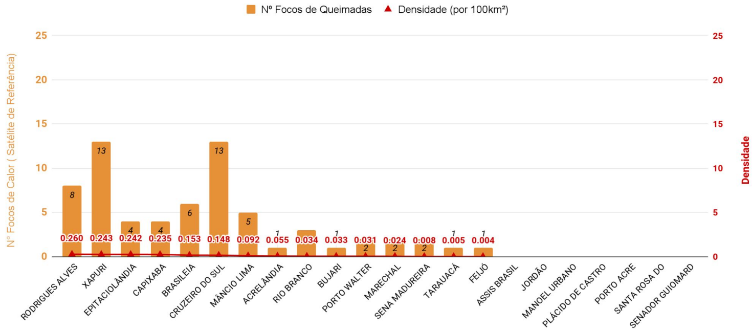
Figura 7 – Ocorrência de focos de queimadas e densidade por km 2 , por município em 01/01/2022 a 07/06/2022 (Satélite de referência AQUA)
