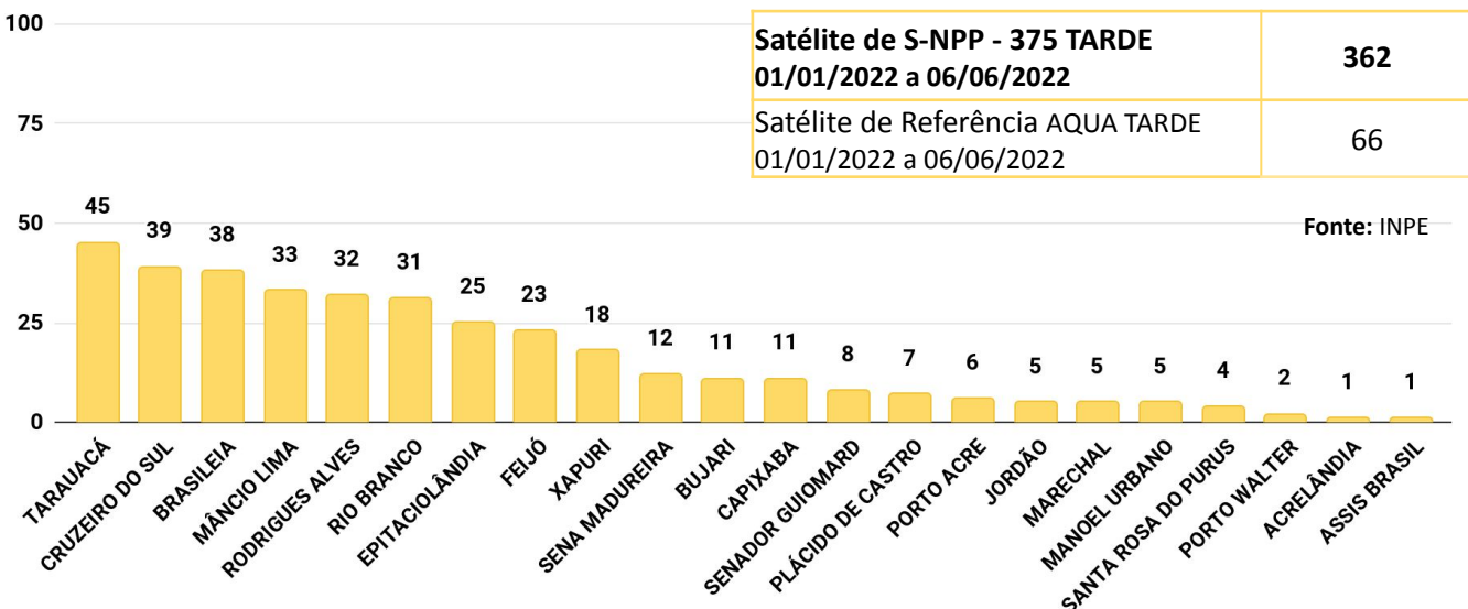
Figura 6 – Distribuição percentual dos focos de queimadas acumulados em 01/01/2022 a 06/06/2022 no estado do Acre (Satélite S-NPP - 375 TARDE)
