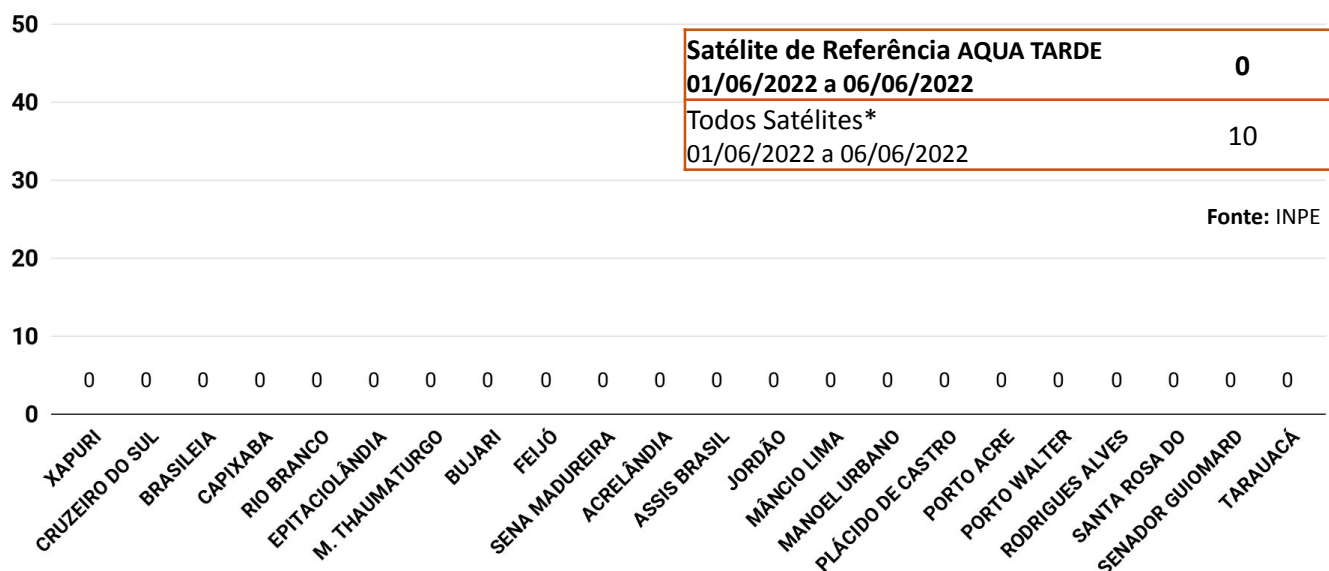
Figura 5 – Distribuição percentual dos focos de queimadas acumulados em 01/06/2022 a 06/06/2022 no estado do Acre (Satélite de Referência AQUA Tarde)
