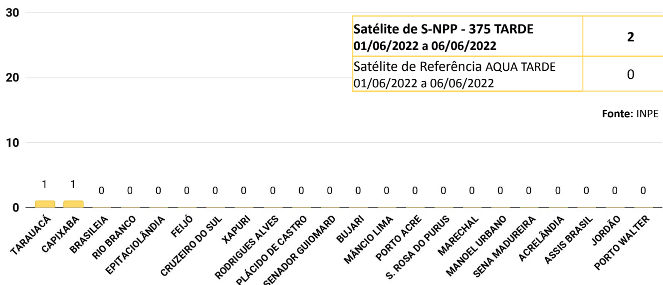
Figura 6 – Distribuição percentual dos focos de queimadas acumulados em 01/06/2022 a 06/06/2022 no estado do Acre (Satélite S-NPP - 375 TARDE)
