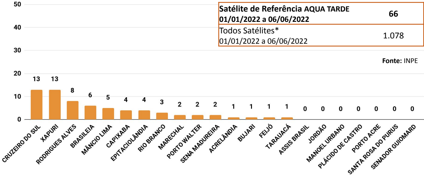
Figura 5 – Distribuição percentual dos focos de queimadas acumulados em 01/01/2022 a 06/06/2022 no estado do Acre (Satélite de Referência AQUA Tarde)
