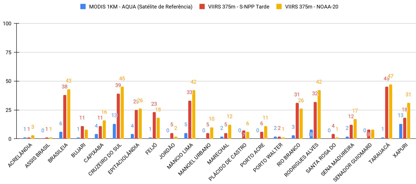
Figura 8 – Distribuição dos focos de queimadas acumulados de 01/01/2022 a 06/06/2022, no Estado do Acre. Satélite de referência AQUA (Barra de cor azul), VIIRS 375m/S-NPP Tarde (Cor vermelha) e VIIRS 375m - NOAA-20 (Cor amarela)
