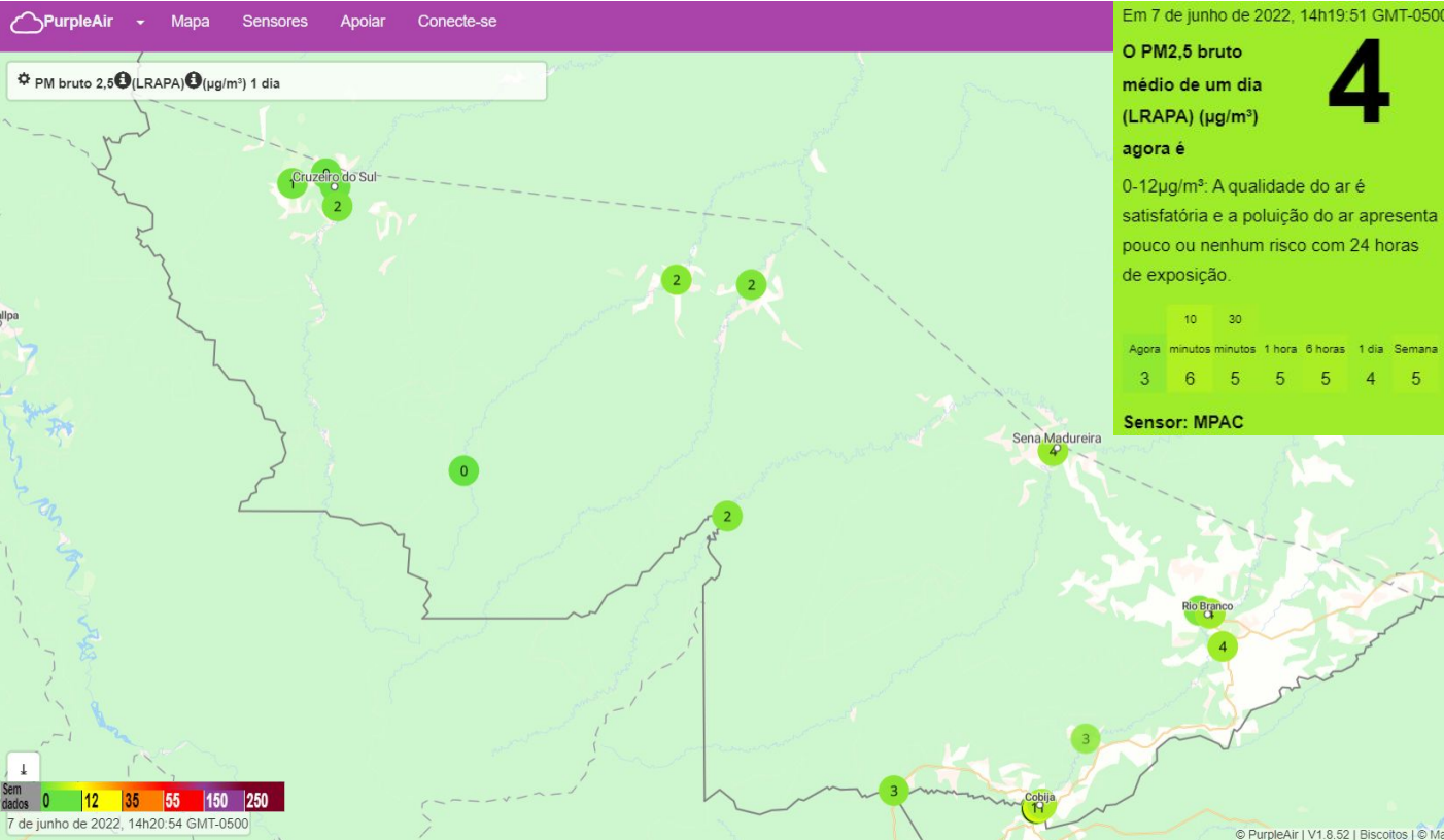
Figura 10 – Concentração de Material Particulado PM 2.5 \mu\text{g}/\text{m}^3 média para dia 07/06/2022.
