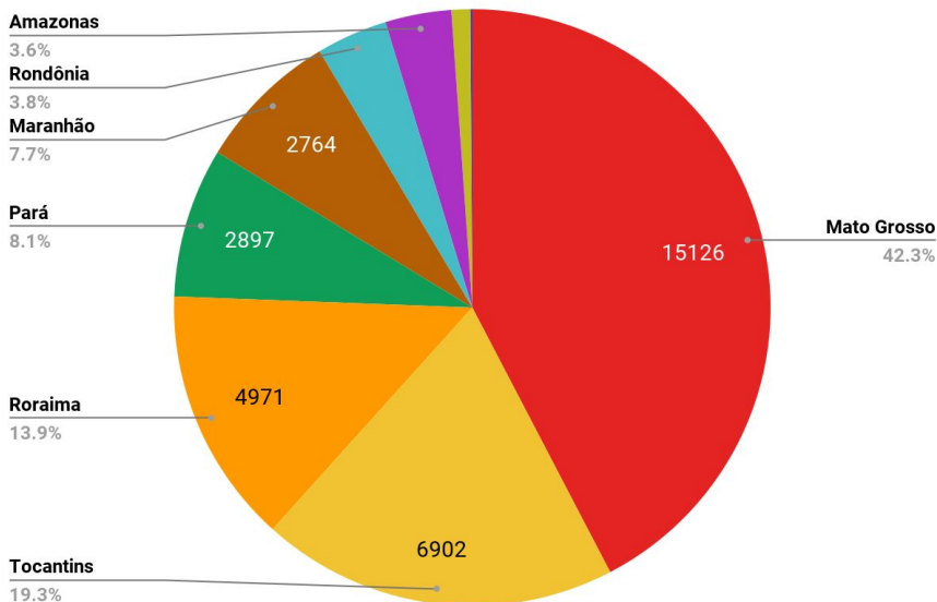
Figura 2 – Distribuição percentual dos focos de queimadas acumulados em 01/01/2022 a 06/06/2022 na Amazônia legal (Satélite S-NPP - 375 TARDE)
