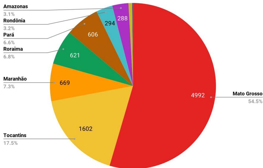
Figura 1 – Distribuição percentual dos focos de queimadas acumulados em 01/01/2022 a 06/06/2022 na Amazônia legal (Satélite de Referência AQUA)
