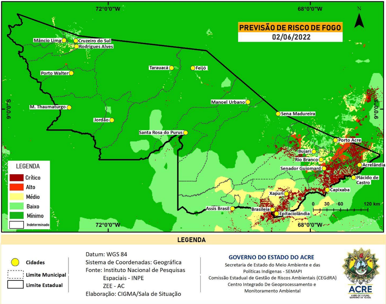
Figura 9 – Risco de Fogo previsto para o estado do Acre para amanhã 02/06/2022
