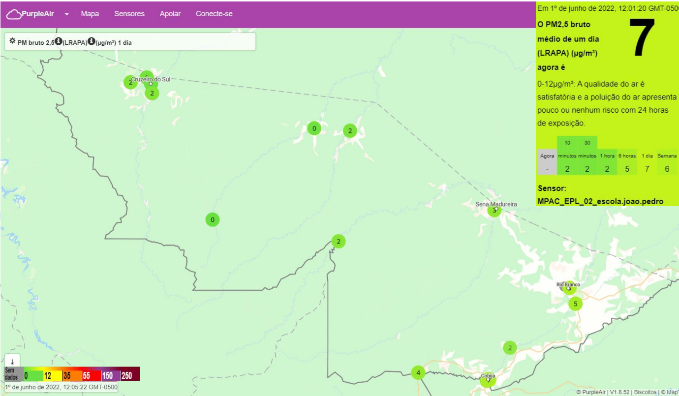
Figura 10 – Concentração de Material Particulado PM 2.5 \mu\text{g}/\text{m}^3 média para dia 01/06/2022.
