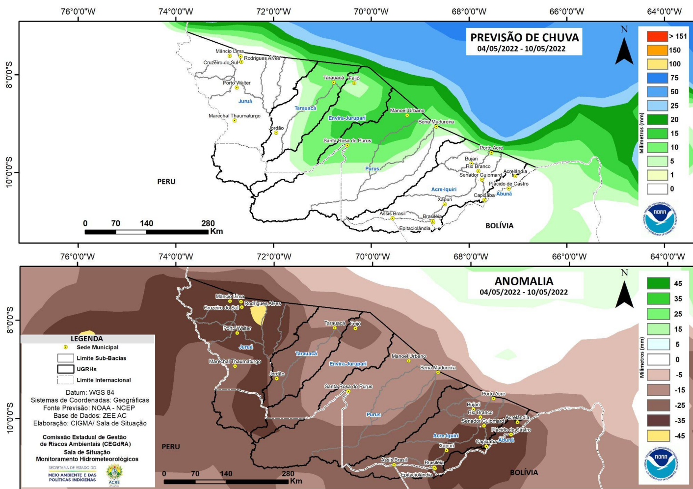
Figura 2: Prognóstico NCEP-GFS/USA.
