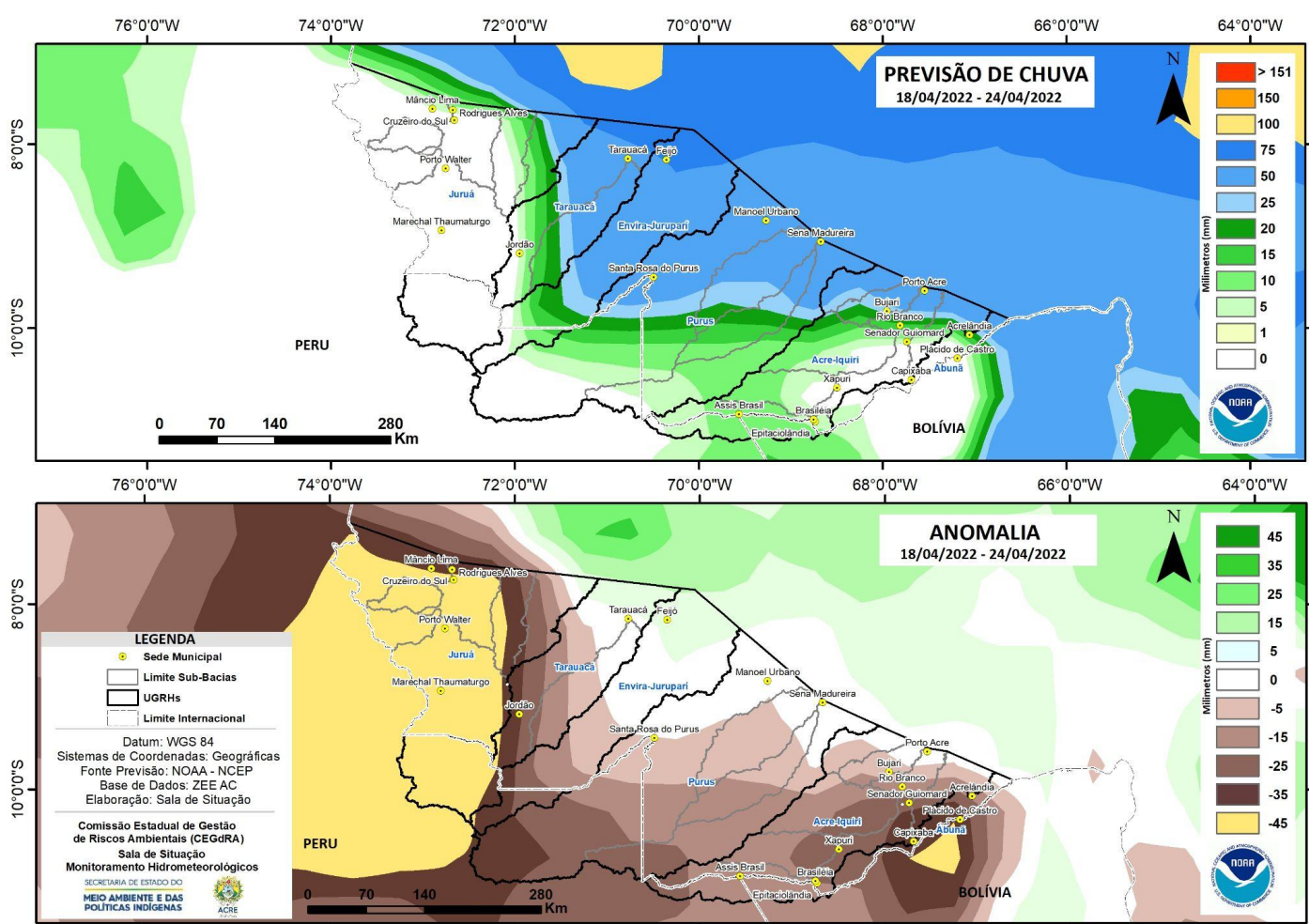
Figura 2: Prognóstico NCEP-GFS/USA.
