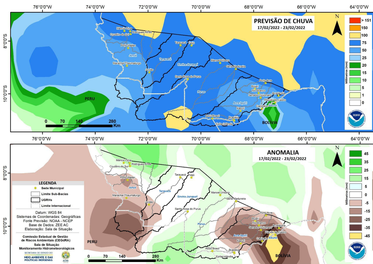
Figura 2: Prognóstico NCEP-GFS/USA.
