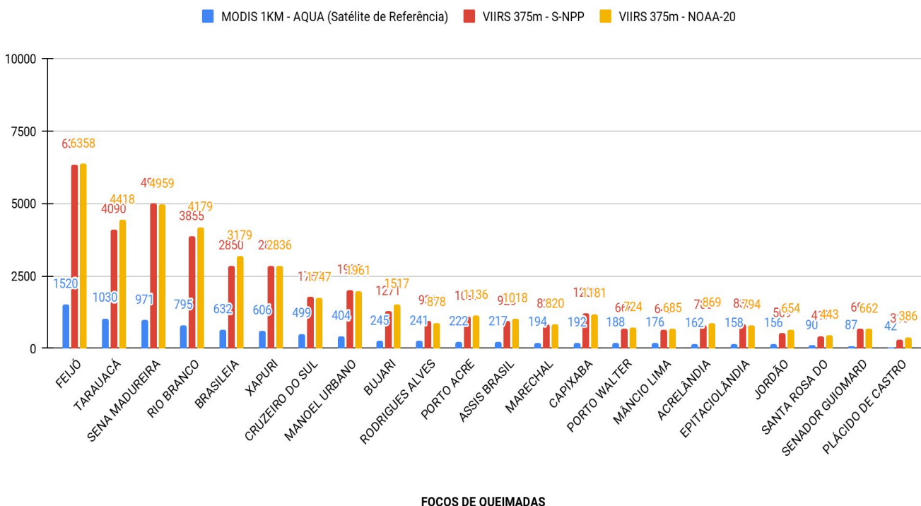
Figura 5 – Distribuição dos focos de queimadas acumulados de 01/01/2021 a 29/11/2021, no Estado do Acre. Satélite de referência AQUA (Barra de cor azul), VIIRS 375m/S-NPP (Cor vermelha) e VIIRS 375m - NOAA-20 (Cor amarela)
