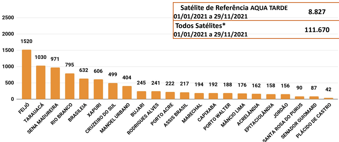
Figura 3 – Distribuição dos focos de queimadas acumulados de 01/01/2021 a 29/11/2021, no Estado do Acre. (Satélite de referência AQUA TARDE)
