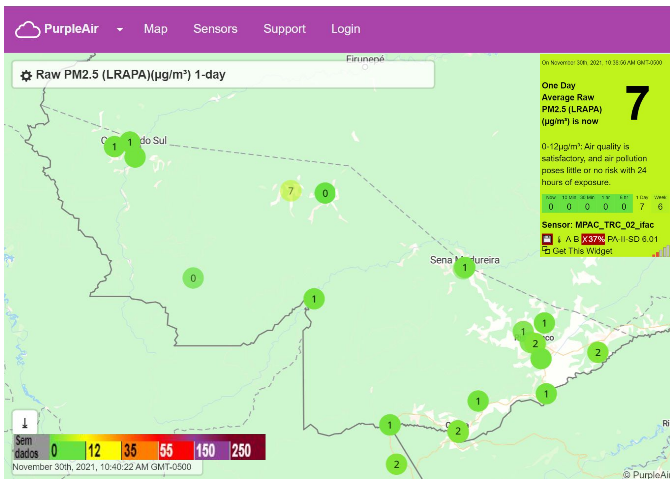
Figura 13 – Concentração de Material Particulado PM 2.5 \mu\text{g}/\text{m}^3 média para dia 30/11/2021.
