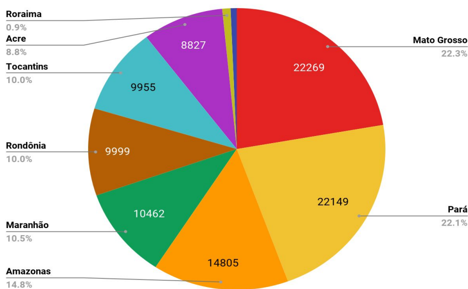
Figura 1 – Distribuição percentual dos focos de queimadas acumulados em 01/01/2021 a 29/11/2021 na Amazônia legal (Satélite de Referência AQUA Tarde)
