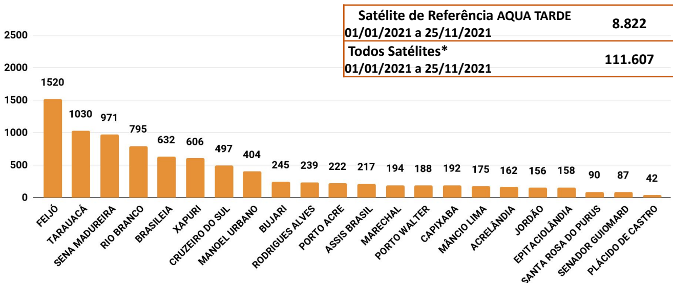
Figura 3 – Distribuição dos focos de queimadas acumulados de 01/01/2021 a 25/11/2021, no Estado do Acre. (Satélite de referência AQUA TARDE)
