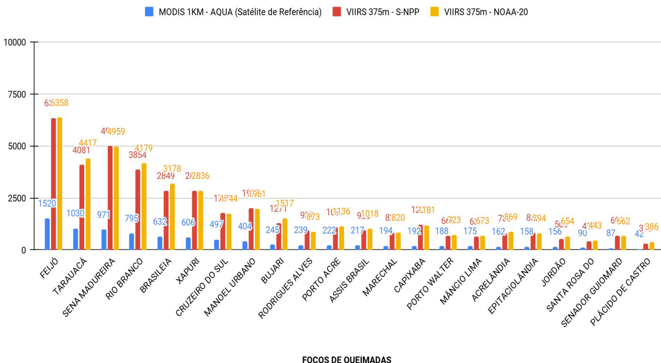
Figura 5 – Distribuição dos focos de queimadas acumulados de 01/01/2021 a 25/11/2021, no Estado do Acre. Satélite de referência AQUA (Barra de cor azul), VIIRS 375m/S-NPP (Cor vermelha) e VIIRS 375m - NOAA-20 (Cor amarela)
