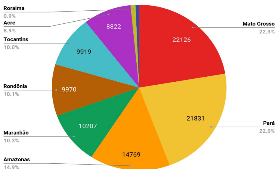
Figura 1 – Distribuição percentual dos focos de queimadas acumulados em 01/01/2021 a 25/11/2021 na Amazônia legal (Satélite de Referência AQUA Tarde)
