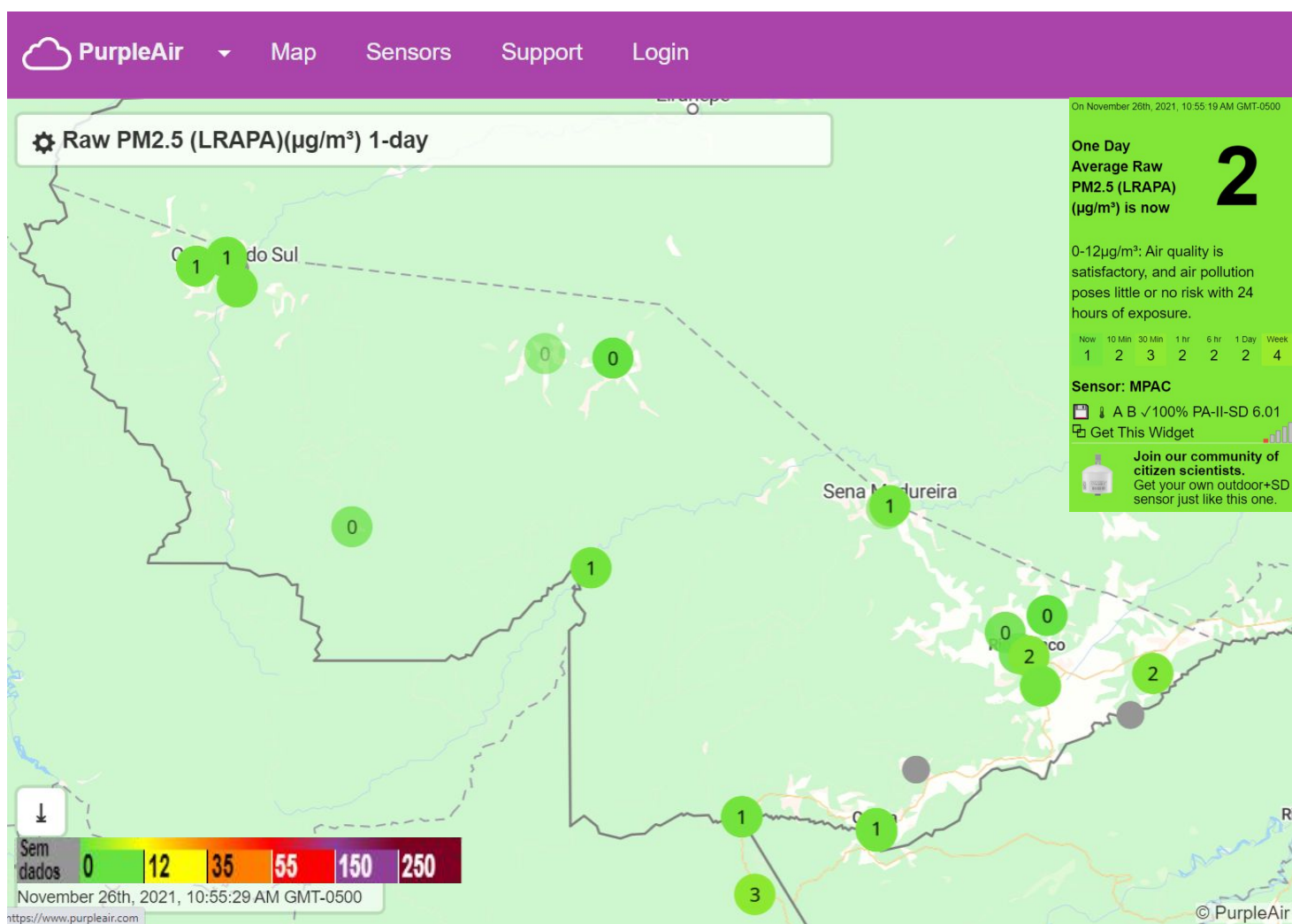
Figura 13 – Concentração de Material Particulado PM 2.5 \mu\text{g}/\text{m}^3 média para dia 26/11/2021.
