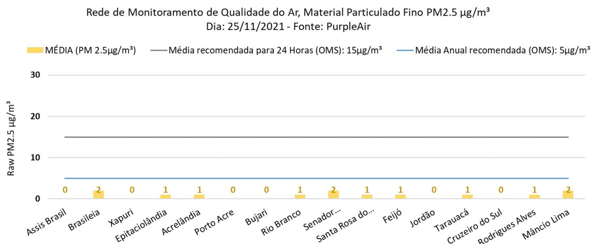
Figura 12 – Valores médios de 25/11/2021 de Material Particulado PM 2.5 \mu\text{g}/\text{m}^3
