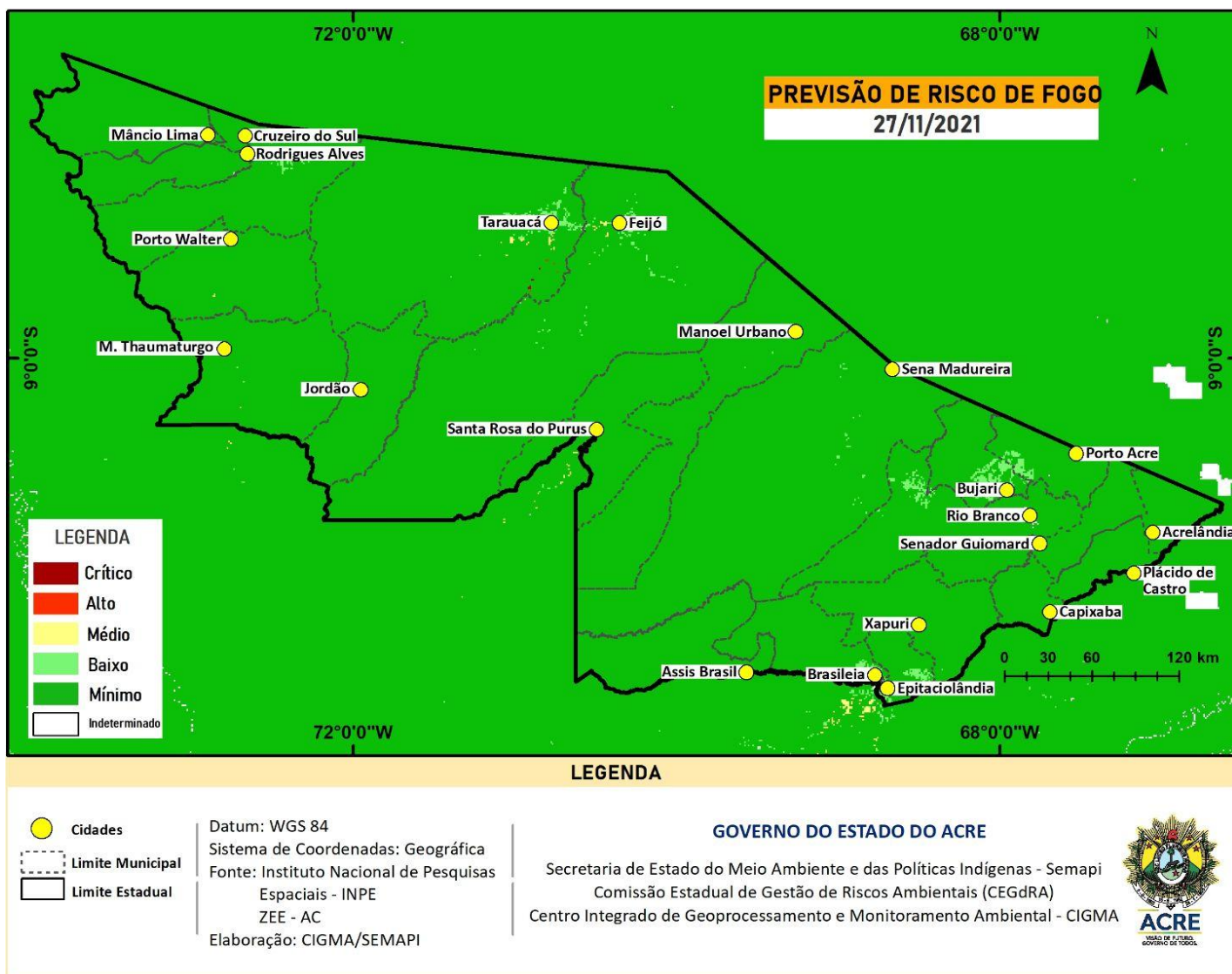
Figura 10 – Risco de Fogo previsto para o estado do Acre para amanhã 27/11/2021
