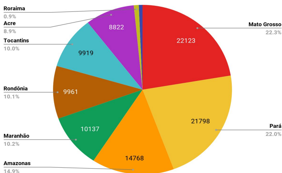
Figura 1 – Distribuição percentual dos focos de queimadas acumulados em 01/01/2021 a 24/11/2021 na Amazônia legal (Satélite de Referência AQUA Tarde)
