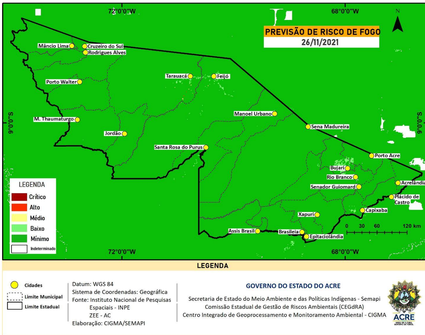
Figura 10 – Risco de Fogo previsto para o estado do Acre para amanhã 26/11/2021
