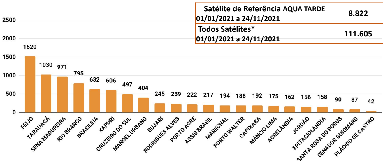
Figura 3 – Distribuição dos focos de queimadas acumulados de 01/01/2021 a 24/11/2021, no Estado do Acre. (Satélite de referência AQUA TARDE)
