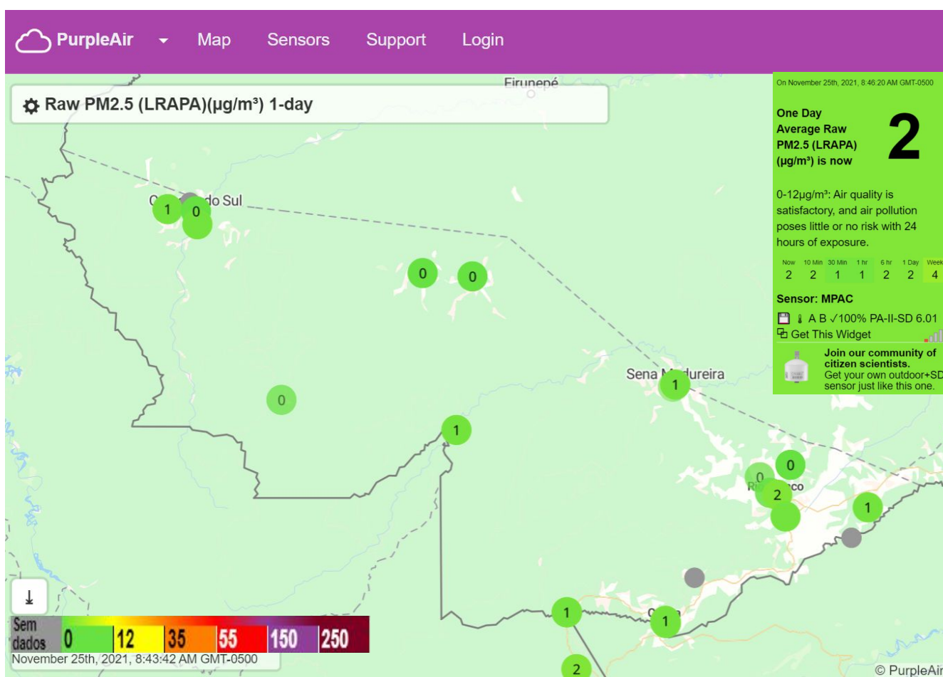
Figura 13 – Concentração de Material Particulado PM 2.5 \mu\text{g}/\text{m}^3 média para dia 25/11/2021.
