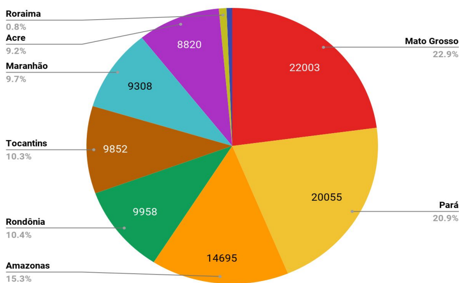
Figura 1 – Distribuição percentual dos focos de queimadas acumulados em 01/01/2021 a 11/11/2021 na Amazônia legal (Satélite de Referência AQUA Tarde)
