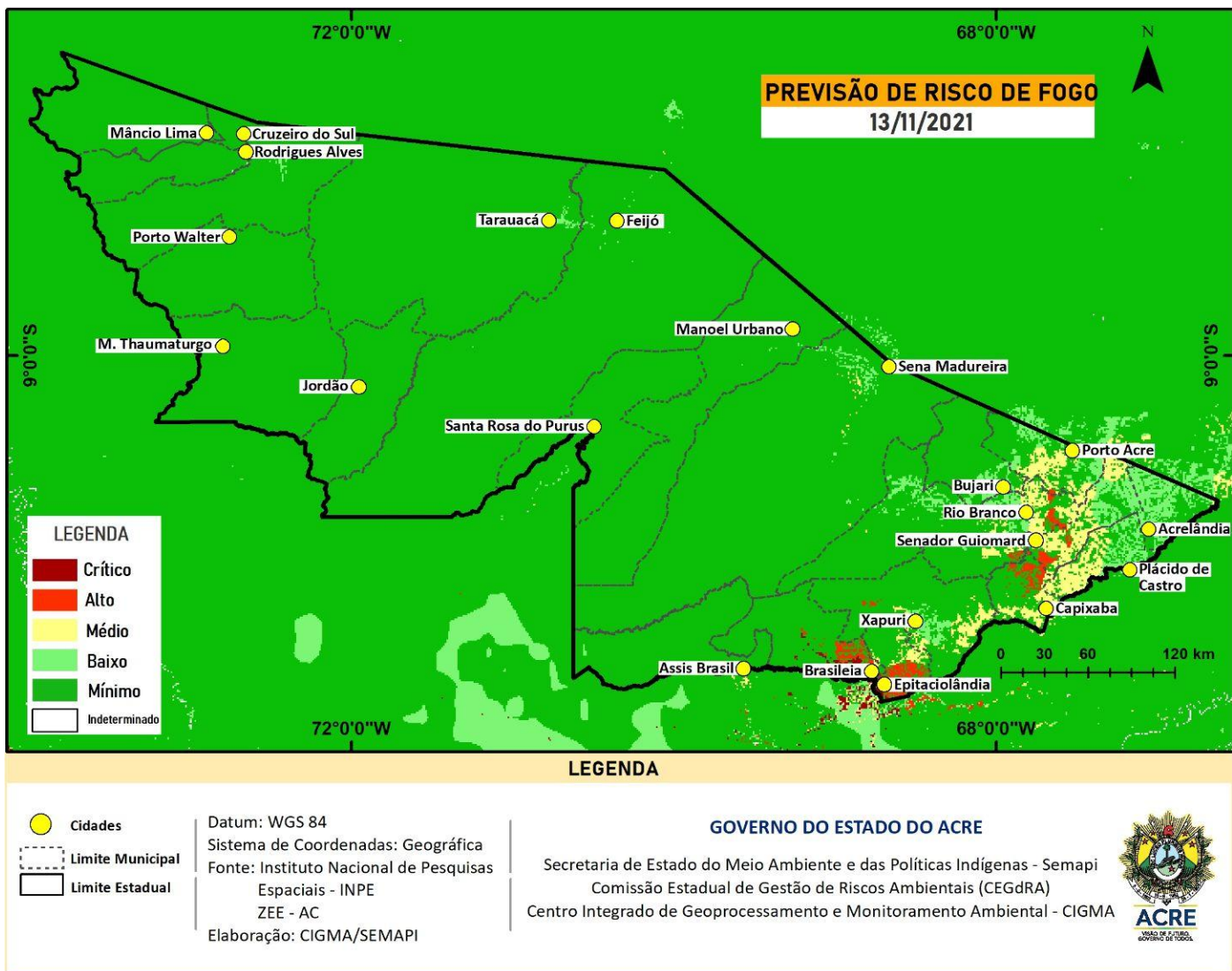
Figura 10 – Risco de Fogo previsto para o estado do Acre para amanhã 13/11/2021
