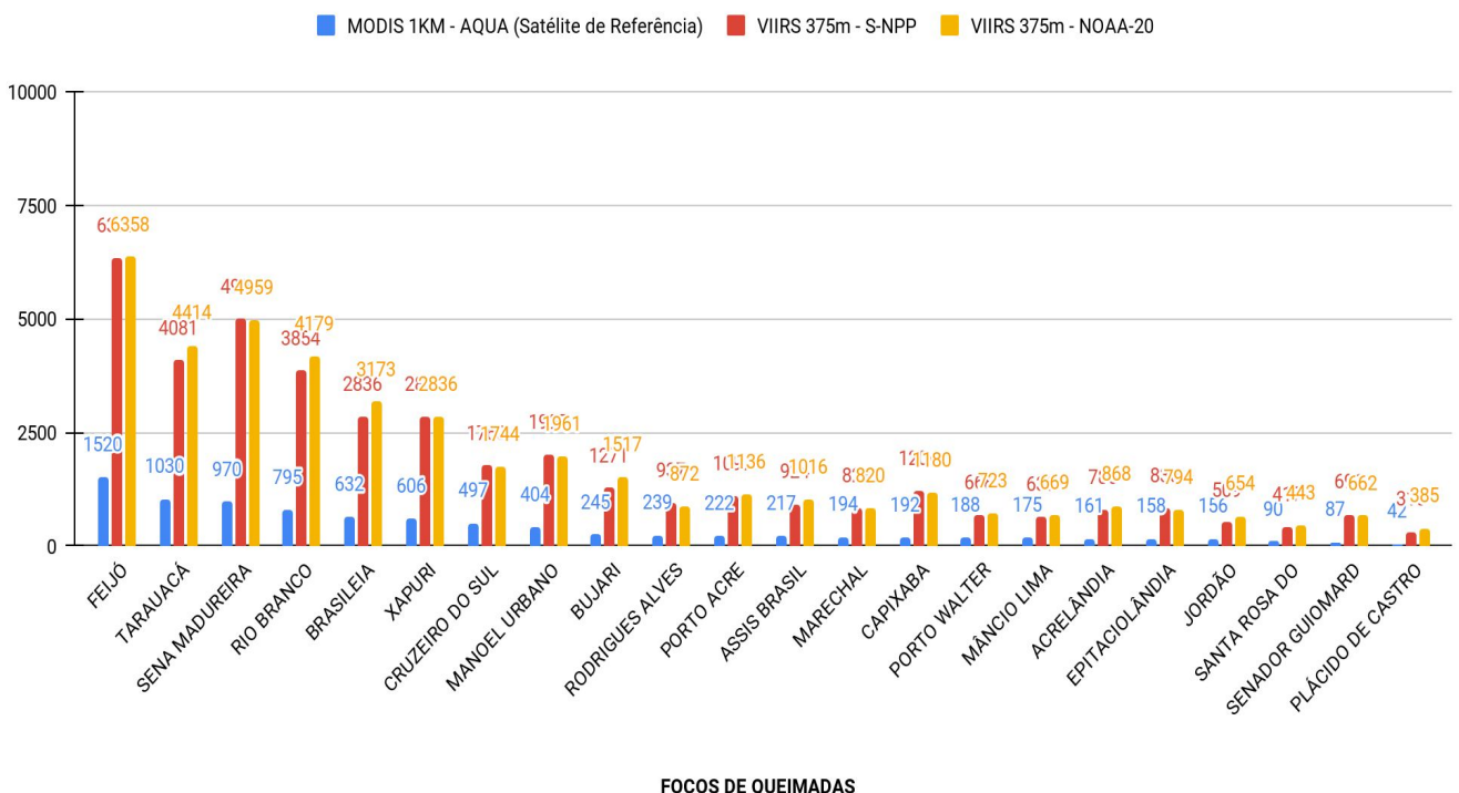
Figura 5 – Distribuição dos focos de queimadas acumulados de 01/01/2021 a 11/11/2021, no Estado do Acre. Satélite de referência AQUA (Barra de cor azul), VIIRS 375m/S-NPP (Cor vermelha) e VIIRS 375m - NOAA-20 (Cor amarela)
