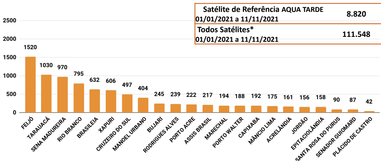
Figura 3 – Distribuição dos focos de queimadas acumulados de 01/01/2021 a 11/11/2021, no Estado do Acre. (Satélite de referência AQUA TARDE)
