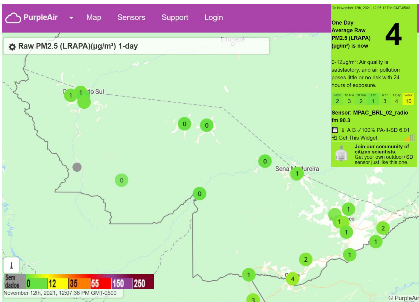
Figura 13 – Concentração de Material Particulado PM 2.5 \mu\text{g}/\text{m}^3 média para dia 12/11/2021.
