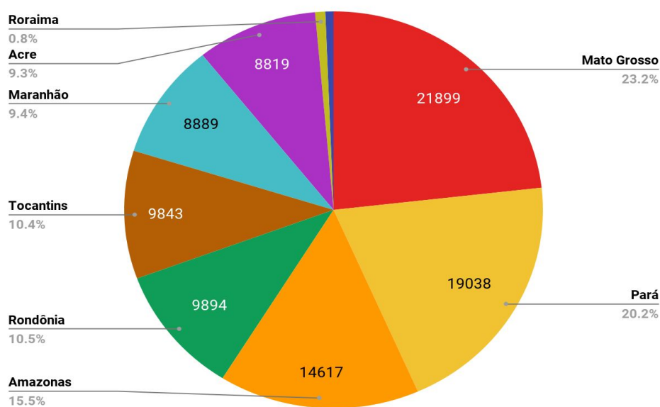
Figura 1 – Distribuição percentual dos focos de queimadas acumulados em 01/01/2021 a 03/11/2021 na Amazônia legal (Satélite de Referência AQUA Tarde)
