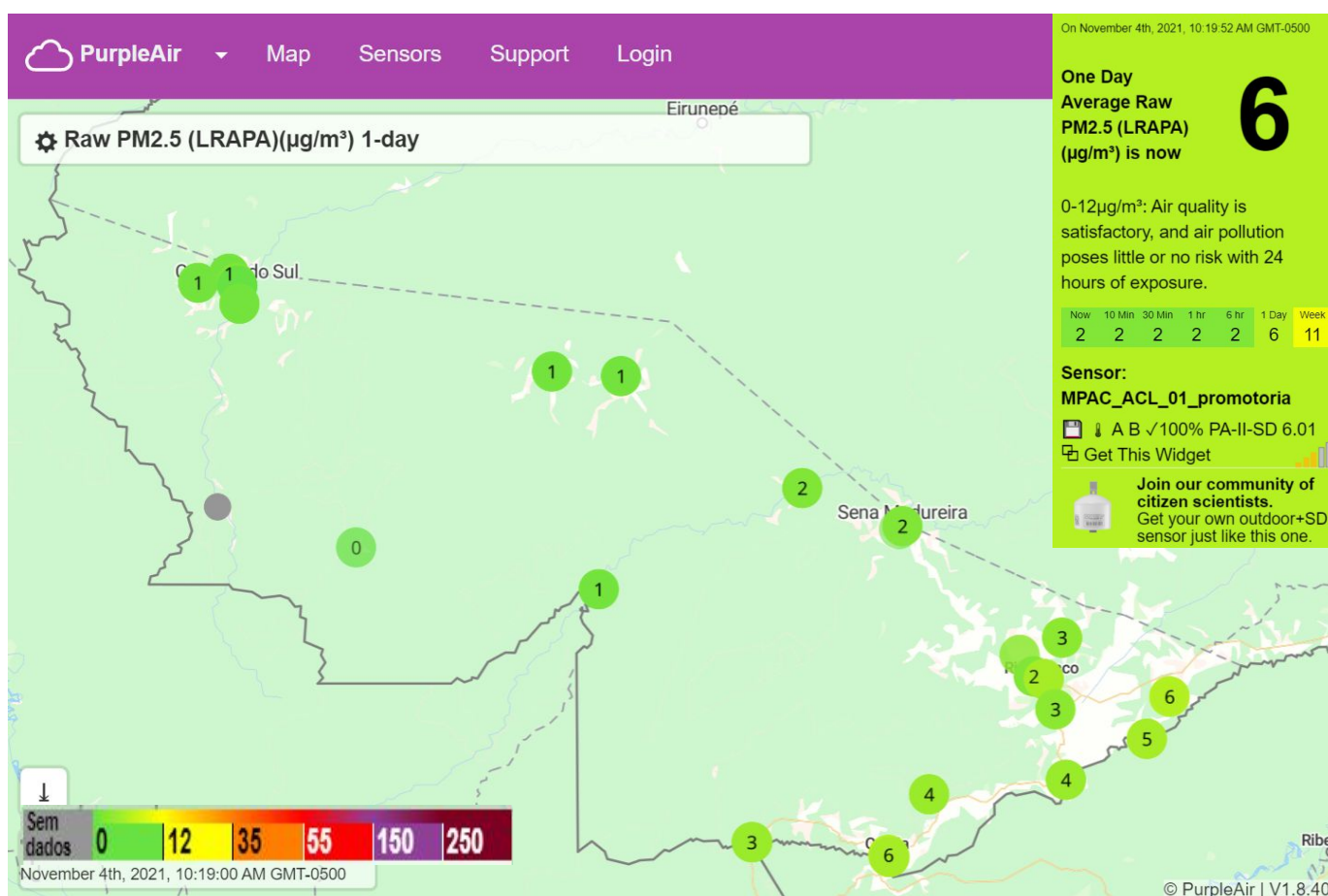
Figura 13 – Concentração de Material Particulado PM 2.5 \mu\text{g}/\text{m}^3 média para dia 04/11/2021.
