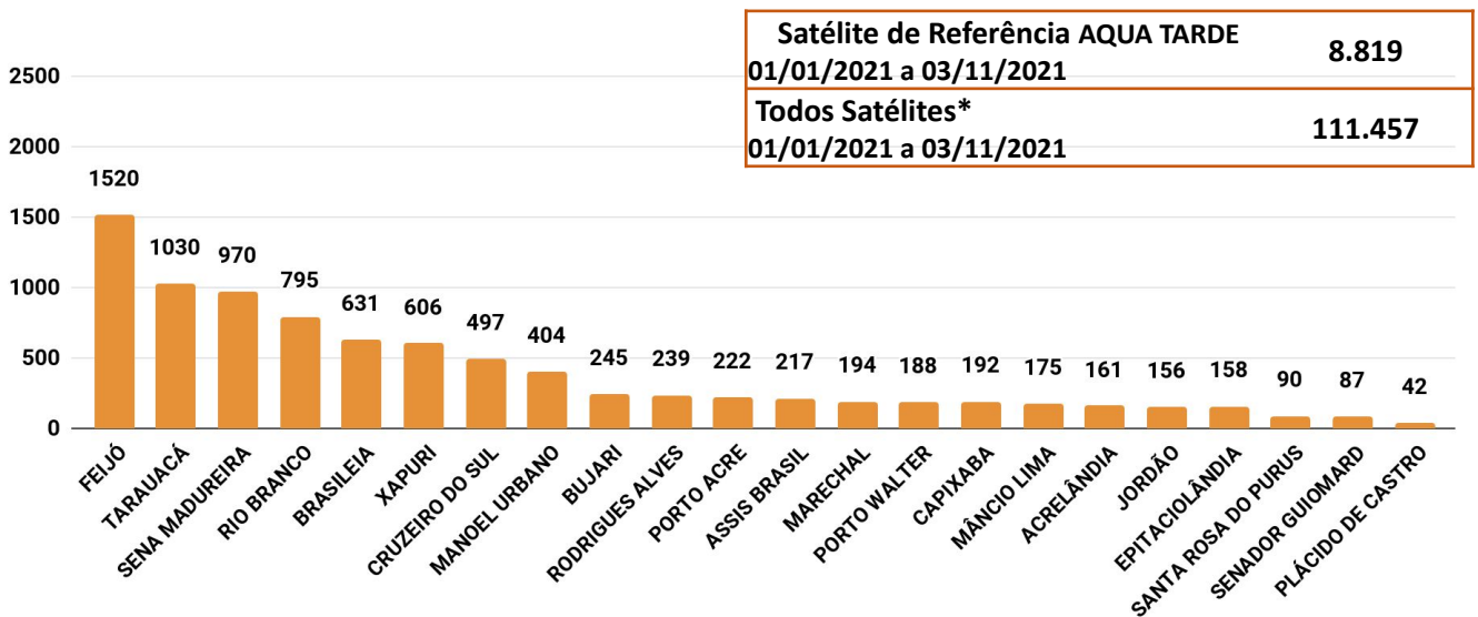
Figura 3 – Distribuição dos focos de queimadas acumulados de 01/01/2021 a 03/11/2021, no Estado do Acre. (Satélite de referência AQUA TARDE)
