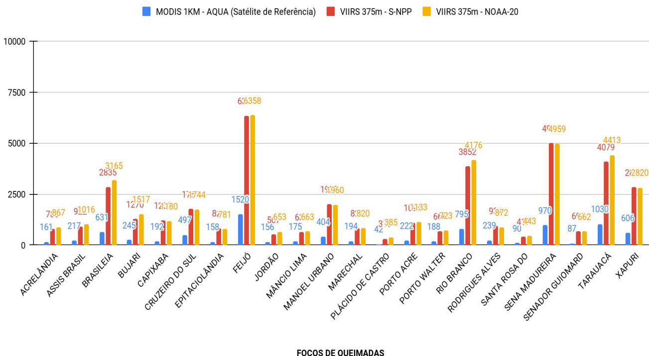
Figura 5 – Distribuição dos focos de queimadas acumulados de 01/01/2021 a 03/11/2021 , no Estado do Acre. Satélite de referência AQUA (Barra de cor azul), VIIRS 375m/S-NPP (Cor vermelha) e VIIRS 375m - NOAA-20 (Cor amarela)
