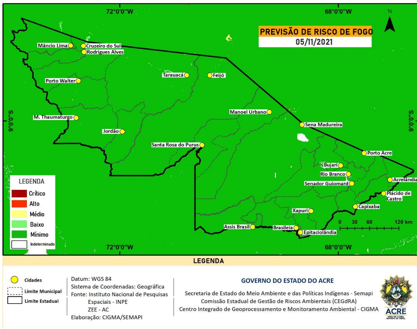
Figura 10 – Risco de Fogo previsto para o estado do Acre para amanhã 05/11/2021
