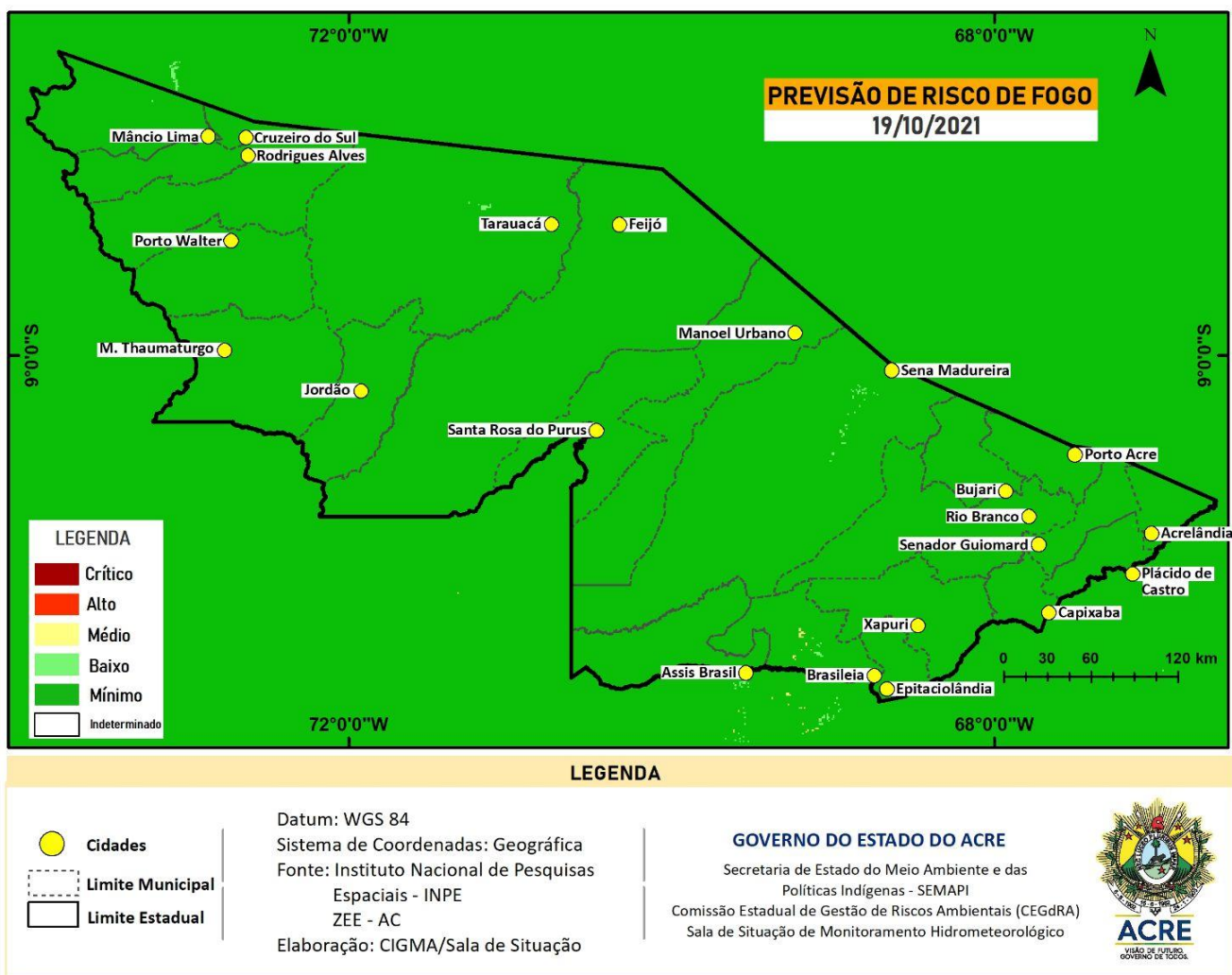
Figura 10 – Risco de Fogo previsto para o estado do Acre para amanhã 19/10/2021
