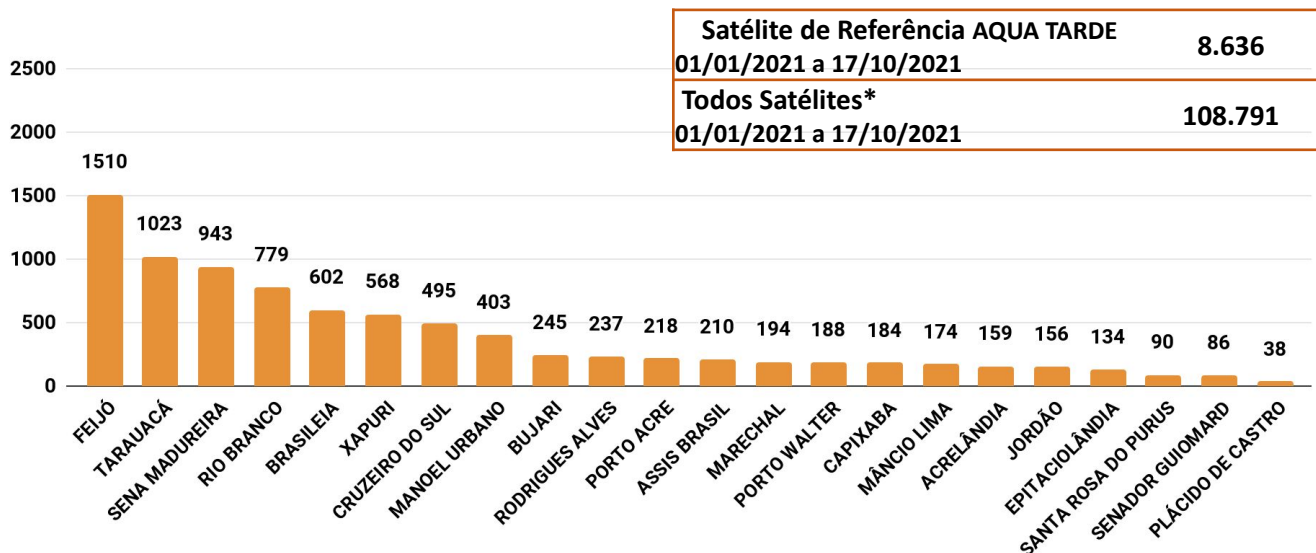
Figura 3 – Distribuição dos focos de queimadas acumulados de 01/01/2021 a 17/10/2021, no Estado do Acre. (Satélite de referência AQUA TARDE)
