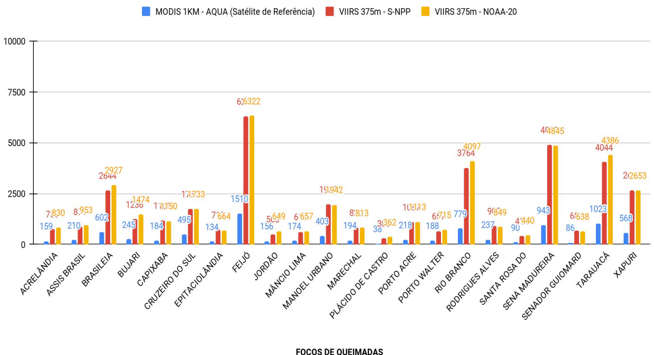
Figura 5 – Distribuição dos focos de queimadas acumulados de 01/01/2021 a 17/10/2021, no Estado do Acre. Satélite de referência AQUA (Barra de cor azul), VIIRS 375m/S-NPP (Cor vermelha) e VIIRS 375m - NOAA-20 (Cor amarela)
