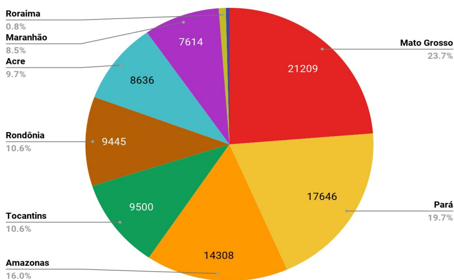
Figura 1 – Distribuição percentual dos focos de queimadas acumulados em 01/01/2021 a 17/10/2021 na Amazônia legal (Satélite de Referência AQUA Tarde)
