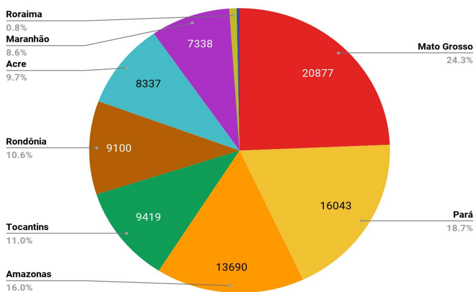
Figura 1 – Distribuição percentual dos focos de queimadas acumulados em 01/01/2021 a 12/10/2021 na Amazônia legal (Satélite de Referência AQUA Tarde)
