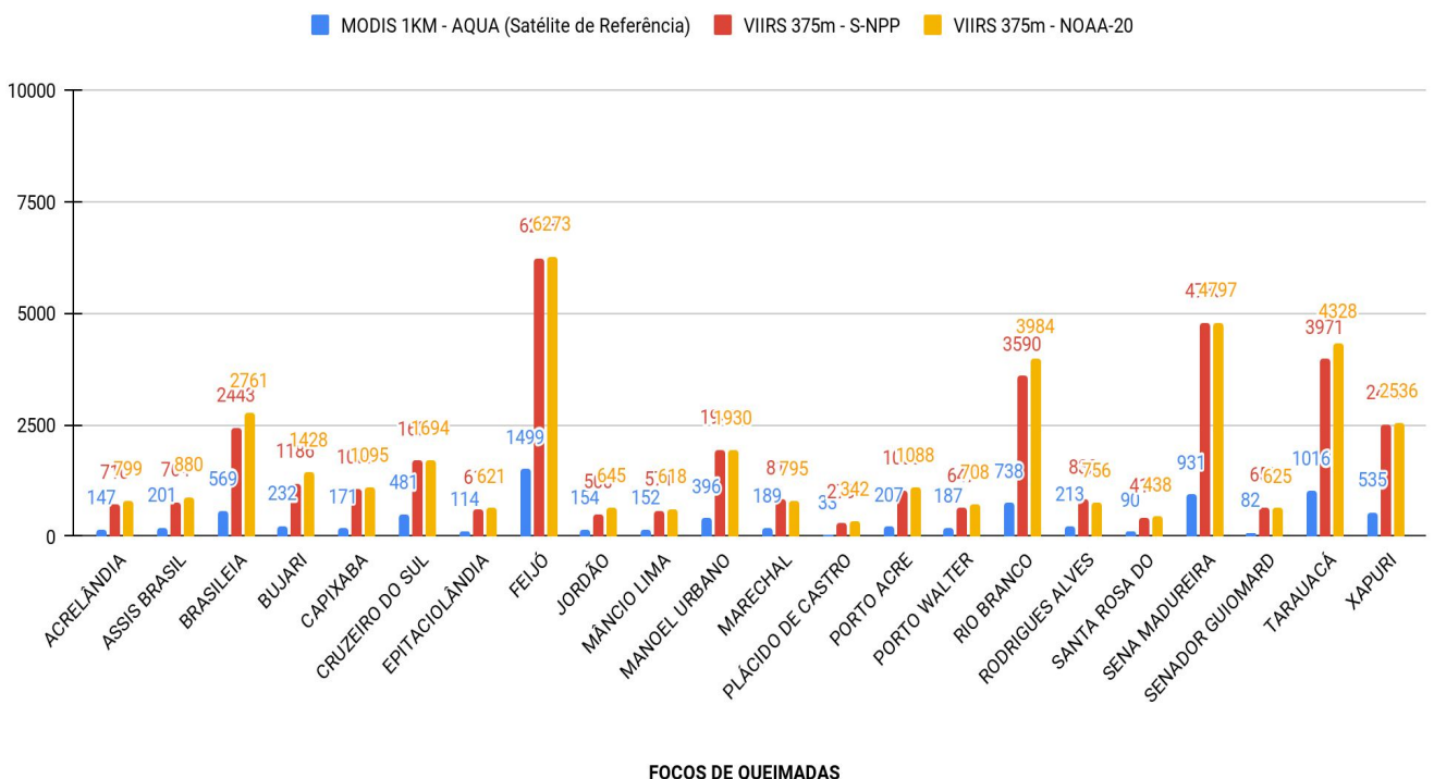
Figura 5 – Distribuição dos focos de queimadas acumulados de 01/01/2021 a 12/10/2021, no Estado do Acre. Satélite de referência AQUA (Barra de cor azul), VIIRS 375m/S-NPP (Cor vermelha) e VIIRS 375m - NOAA-20 (Cor amarela)
