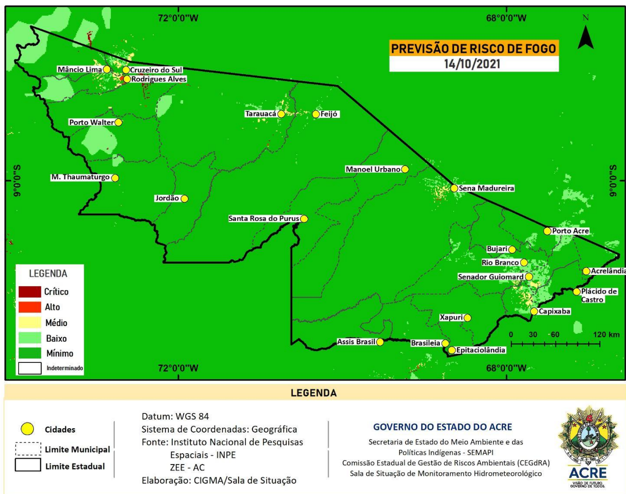
Figura 8 – Risco de Fogo previsto para o estado do Acre para amanhã 14/10/2021
