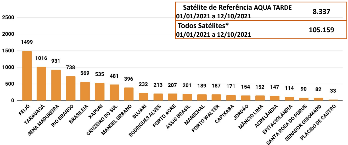
Figura 3 – Distribuição dos focos de queimadas acumulados de 01/01/2021 a 12/10/2021, no Estado do Acre. (Satélite de referência AQUA TARDE)
