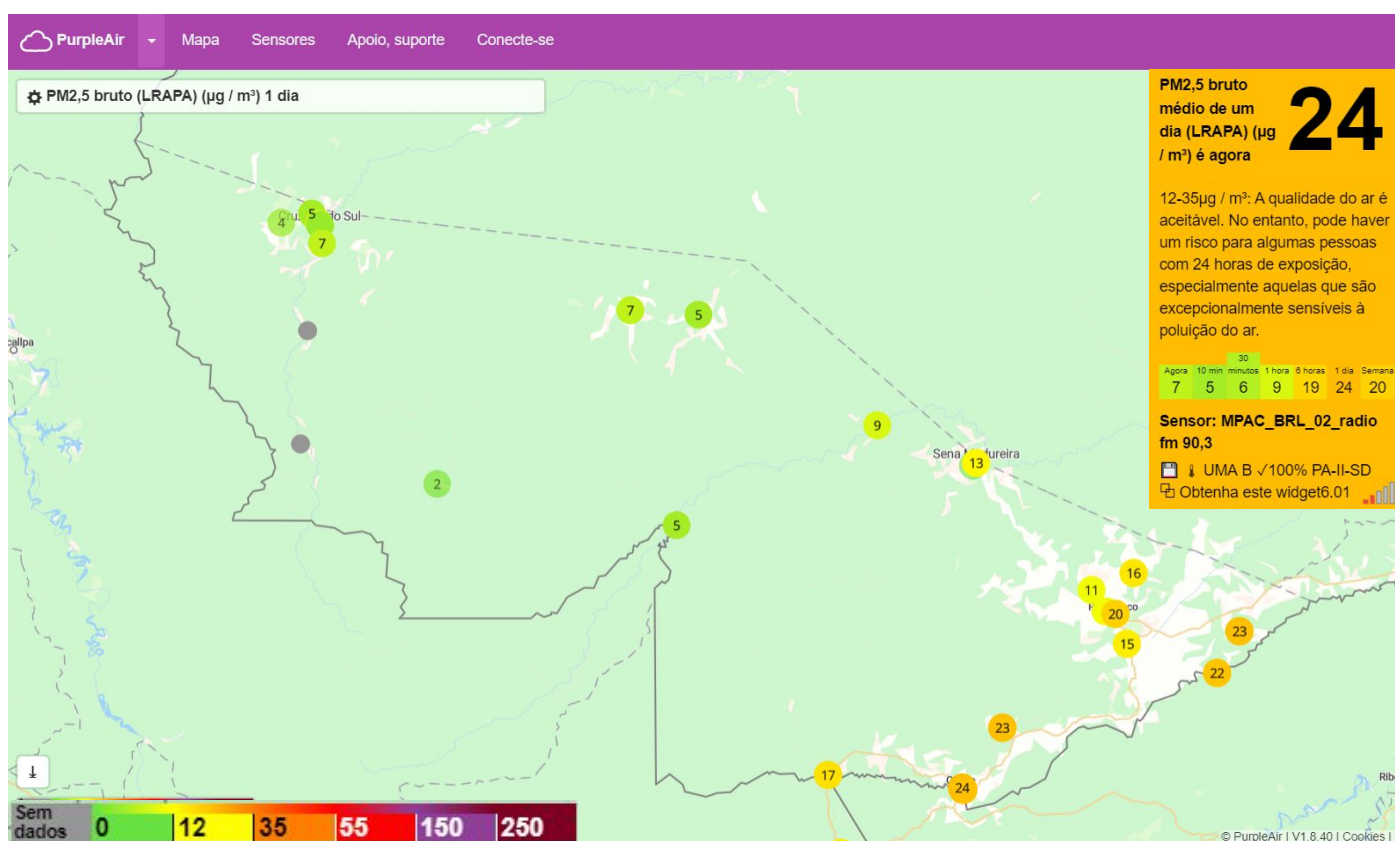
Figura 11 – Concentração de Material Particulado PM 2.5 \mu\text{g}/\text{m}^3 média para dia 13/10/2021.
