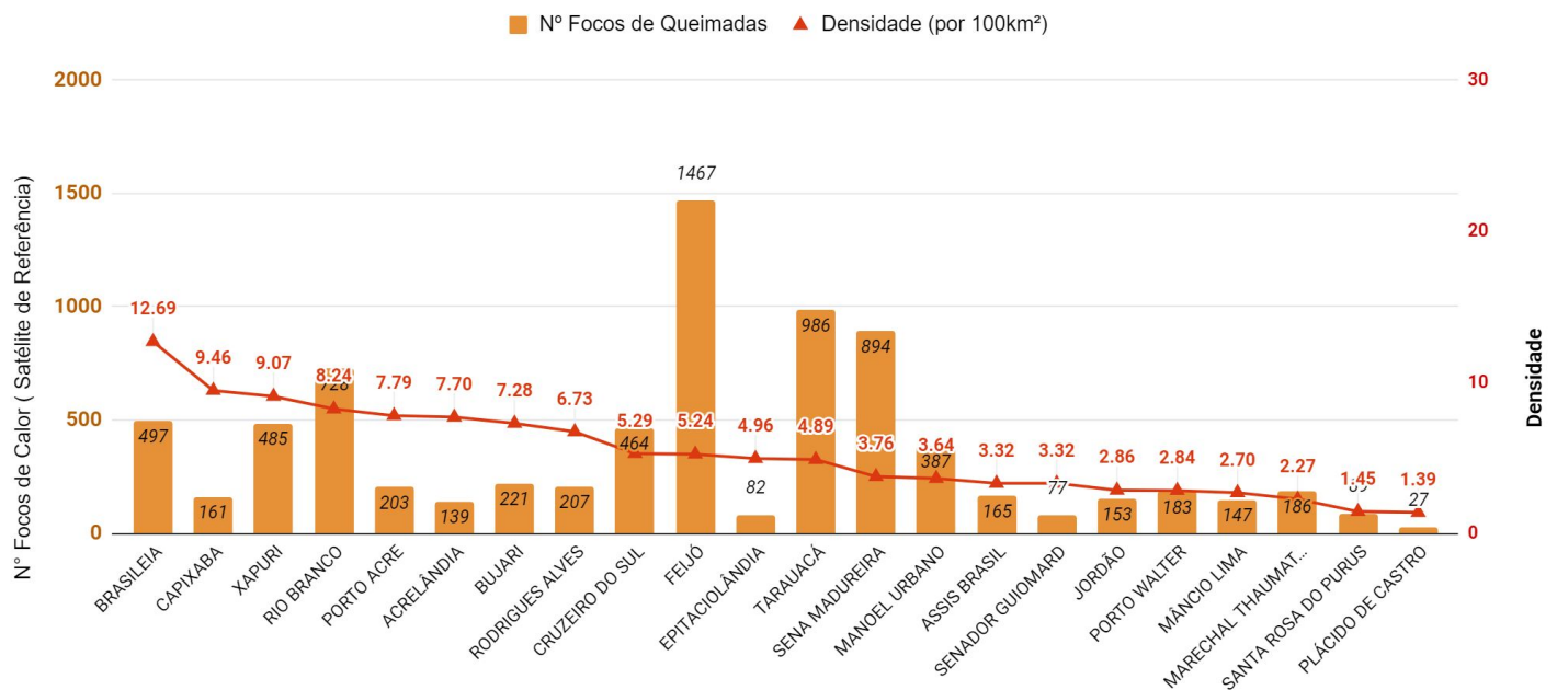
Figura 6 – Ocorrência de focos de queimadas e densidade por km 2 , por município em 01/01/2021 a 03/10/2021 (Satélite de referência AQUA)
