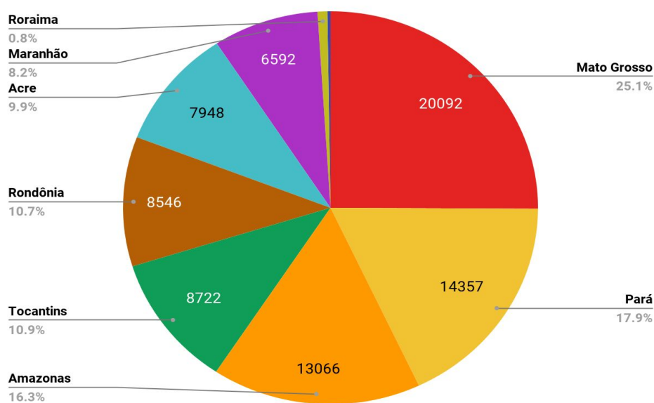
Figura 1 – Distribuição percentual dos focos de queimadas acumulados em 01/01/2021 a 03/10/2021 na Amazônia legal (Satélite de Referência AQUA Tarde)
