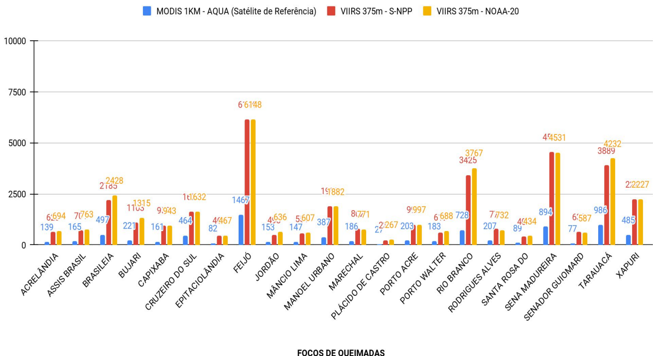
Figura 5 – Distribuição dos focos de queimadas acumulados de 01/01/2021 a 03/10/2021 , no Estado do Acre. Satélite de referência AQUA (Barra de cor azul), VIIRS 375m/S-NPP (Cor vermelha) e VIIRS 375m - NOAA-20 (Cor amarela)
