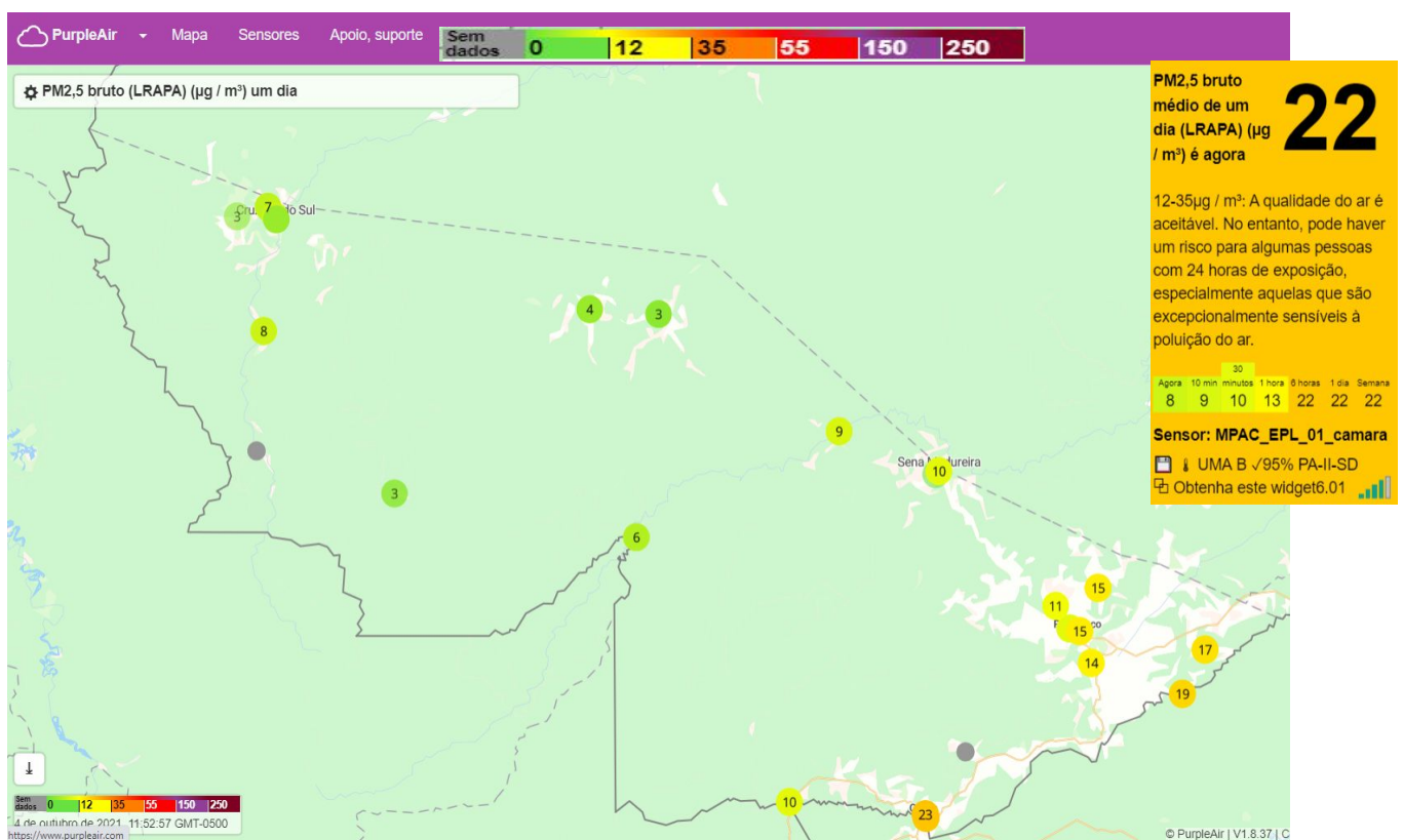
Figura 11 – Concentração de Material Particulado PM 2.5 \mu\text{g}/\text{m}^3 média para dia 04/10/2021.
