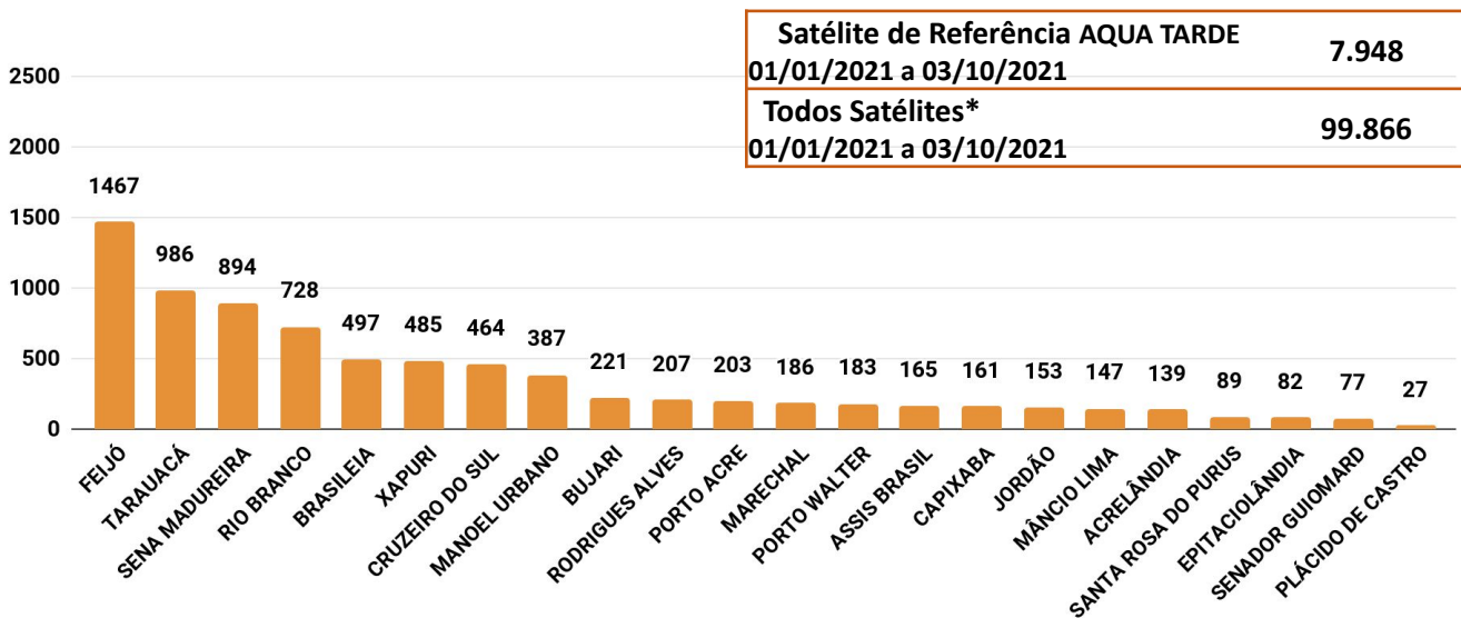
Figura 3 – Distribuição dos focos de queimadas acumulados de 01/01/2021 a 03/10/2021, no Estado do Acre. (Satélite de referência AQUA TARDE)
