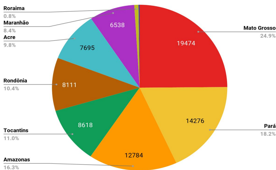
Figura 1 – Distribuição percentual dos focos de queimadas acumulados em 01/01/2021 a 30/09/2021 na Amazônia legal (Satélite de Referência AQUA Tarde)
