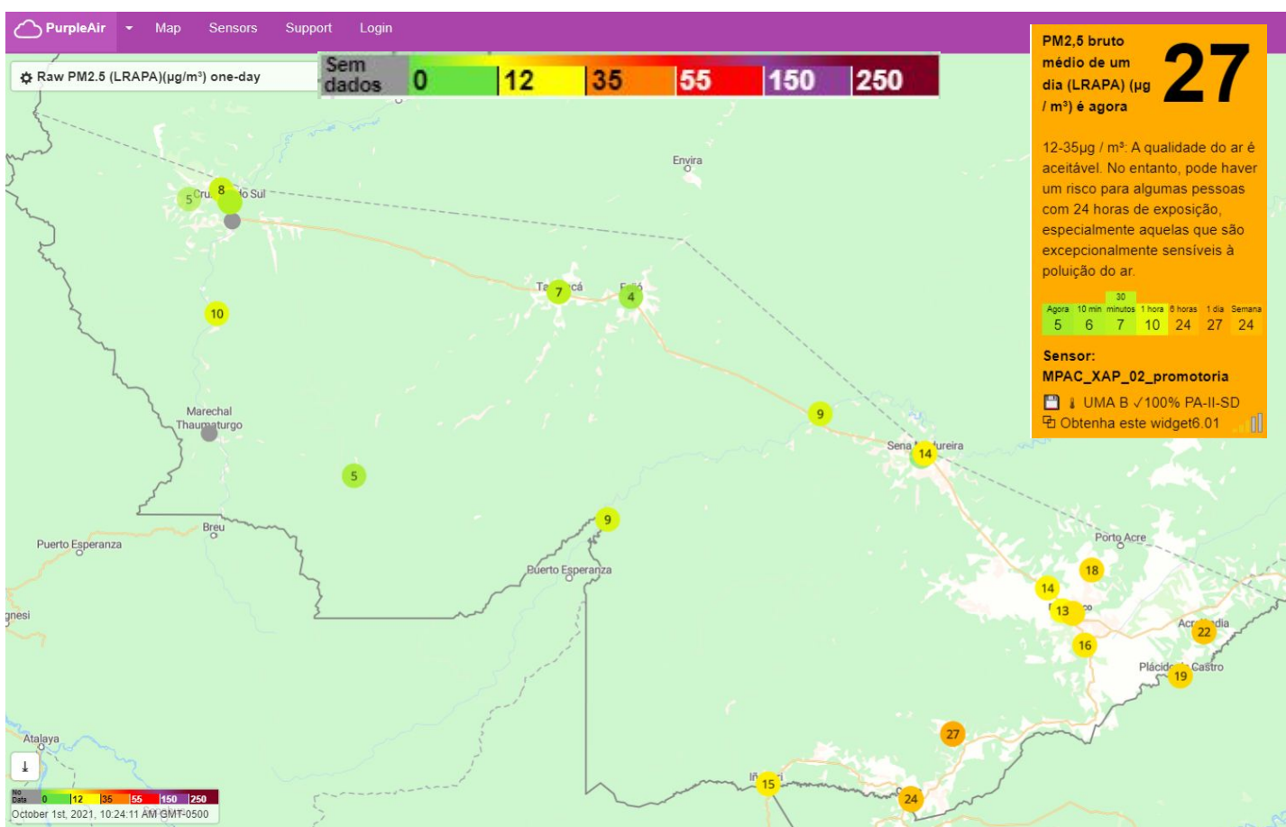
Figura 11 – Concentração de Material Particulado PM 2.5 \mu\text{g}/\text{m}^3 média para dia 01/10/2021.
