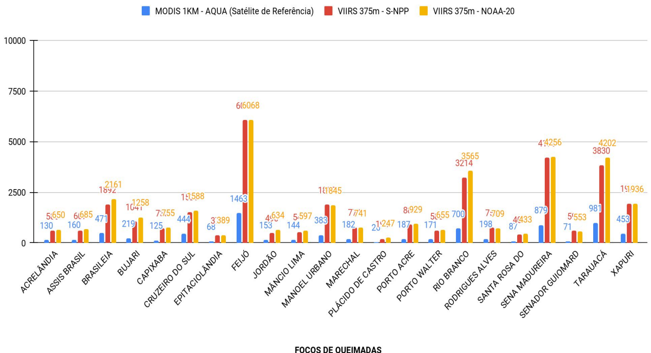
Figura 5 – Distribuição dos focos de queimadas acumulados de 01/01/2021 a 30/09/2021 , no Estado do Acre. Satélite de referência AQUA (Barra de cor azul), VIIRS 375m/S-NPP (Cor vermelha) e VIIRS 375m - NOAA-20 (Cor amarela)
