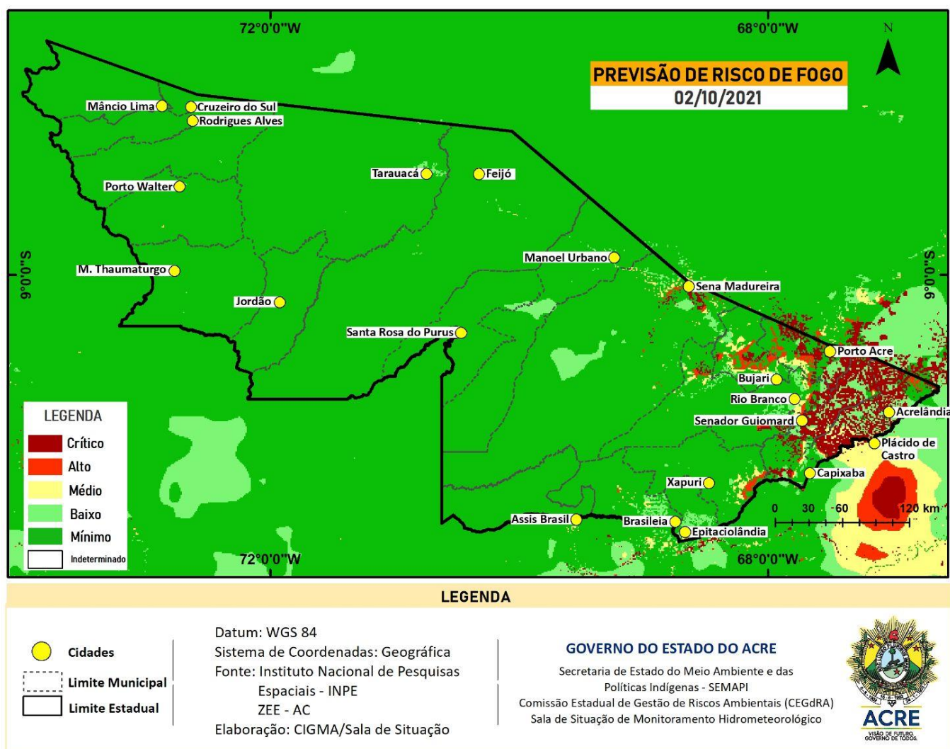
Figura 8 – Risco de Fogo previsto para o estado do Acre para amanhã 02/10/2021
