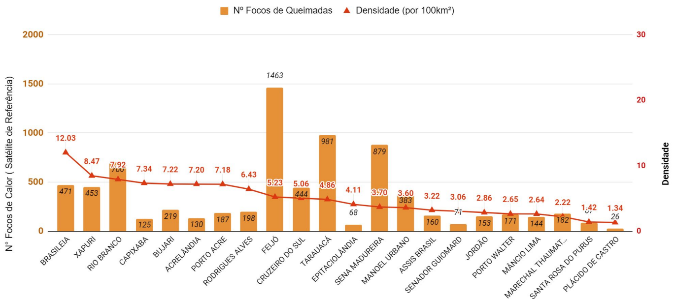
Figura 6 – Ocorrência de focos de queimadas e densidade por km 2 , por município em 01/01/2021 a 30/09/2021 (Satélite de referência AQUA)
