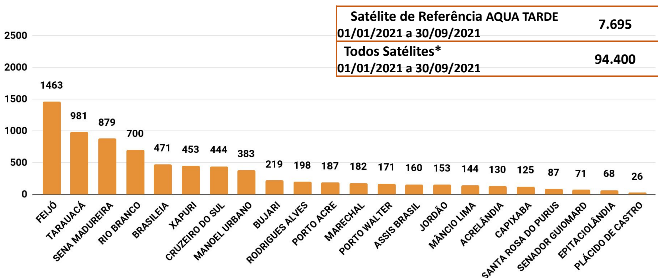
Figura 3 – Distribuição dos focos de queimadas acumulados de 01/01/2021 a 30/09/2021, no Estado do Acre. (Satélite de referência AQUA TARDE)
