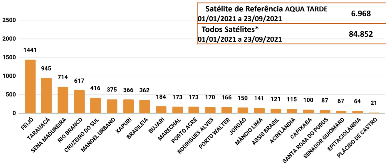
Figura 3 – Distribuição dos focos de queimadas acumulados de 01/01/2021 a 23/09/2021, no Estado do Acre. (Satélite de referência AQUA TARDE)
