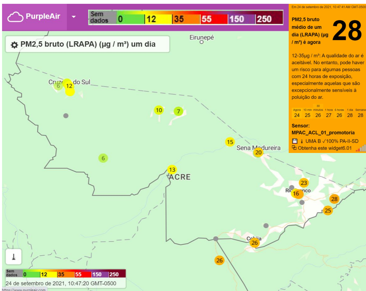
Figura 11 – Concentração de Material Particulado PM 2.5 \mu\text{g}/\text{m}^3 média para dia 24/09/2021.
