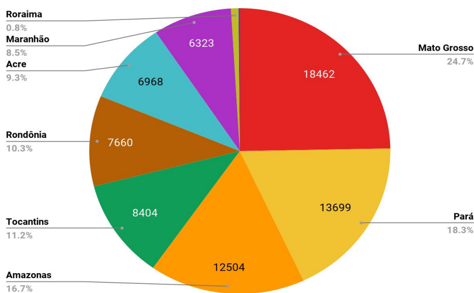
Figura 1 – Distribuição percentual dos focos de queimadas acumulados em 01/01/2021 a 23/09/2021 na Amazônia legal (Satélite de Referência AQUA Tarde)
