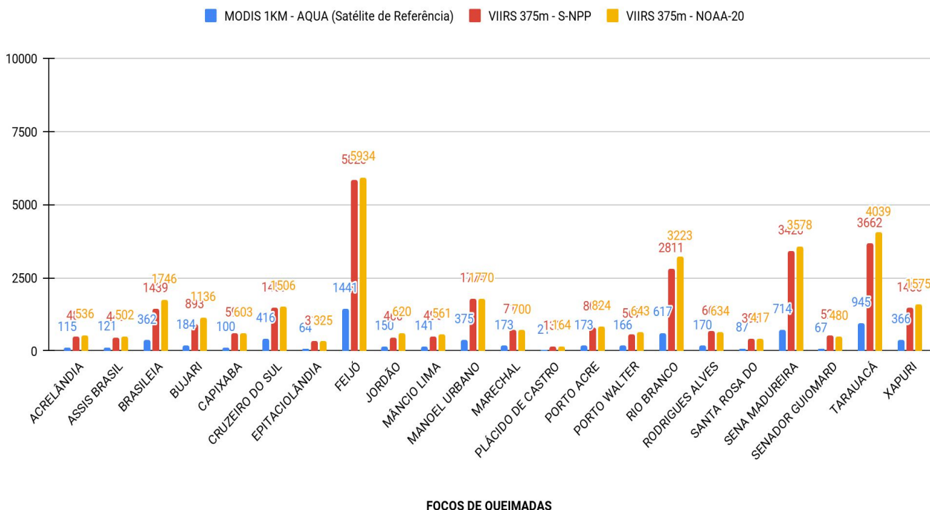
Figura 5 – Distribuição dos focos de queimadas acumulados de 01/01/2021 a 23/09/2021 , no Estado do Acre. Satélite de referência AQUA (Barra de cor azul), VIIRS 375m/S-NPP (Cor vermelha) e VIIRS 375m - NOAA-20 (Cor amarela)
