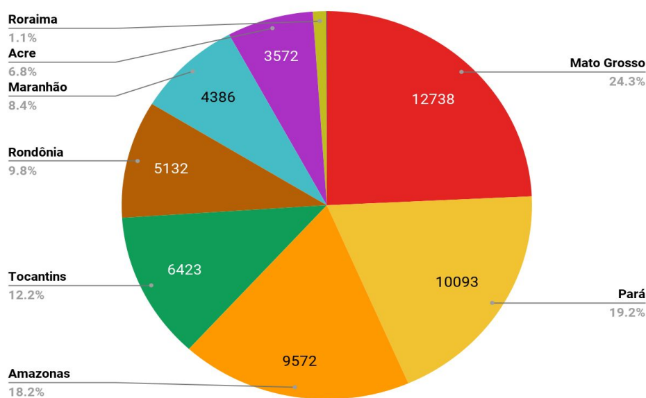
Figura 1 – Distribuição percentual dos focos de queimadas acumulados em 01/01/2021 a 26/08/2021 na Amazônia legal (Satélite de Referência AQUA Tarde)
