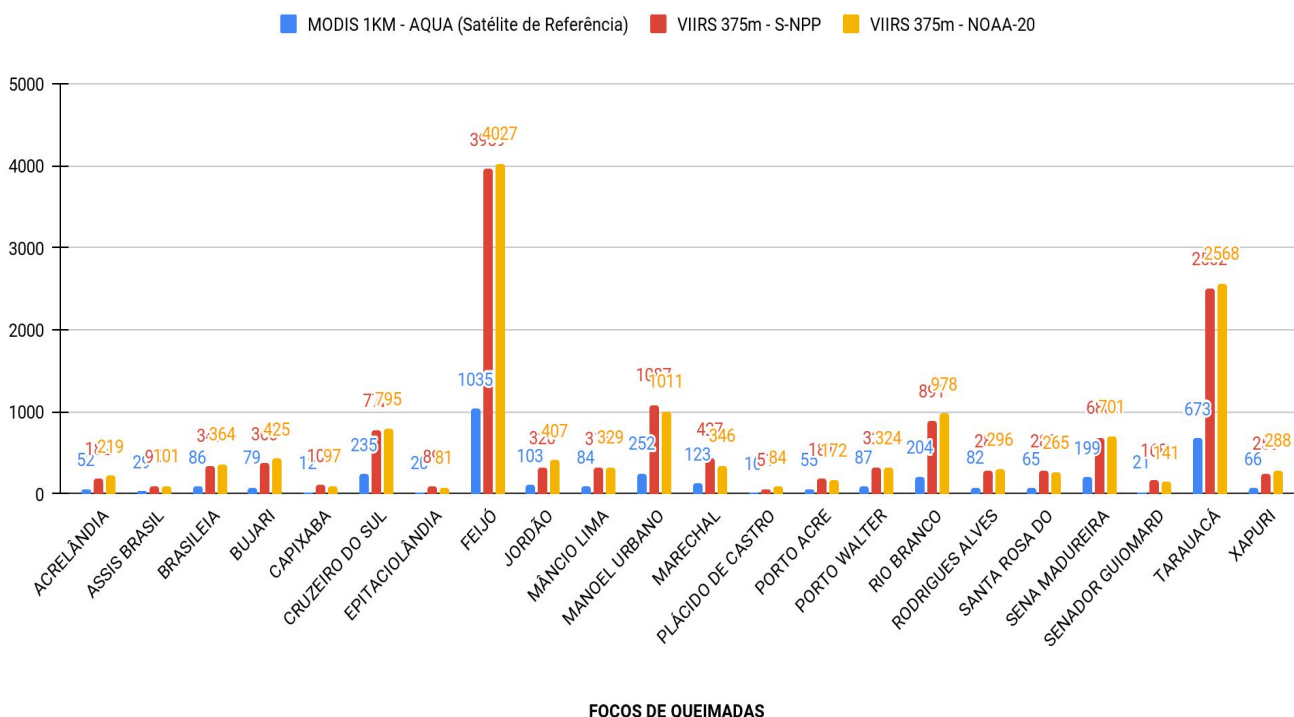
Figura 5 – Distribuição dos focos de queimadas acumulados de 01/01/2021 a 26/08/2021 , no Estado do Acre. Satélite de referência AQUA (Barra de cor azul), VIIRS 375m/S-NPP (Cor vermelha) e VIIRS 375m/NOAA-20 (Cor amarela)
