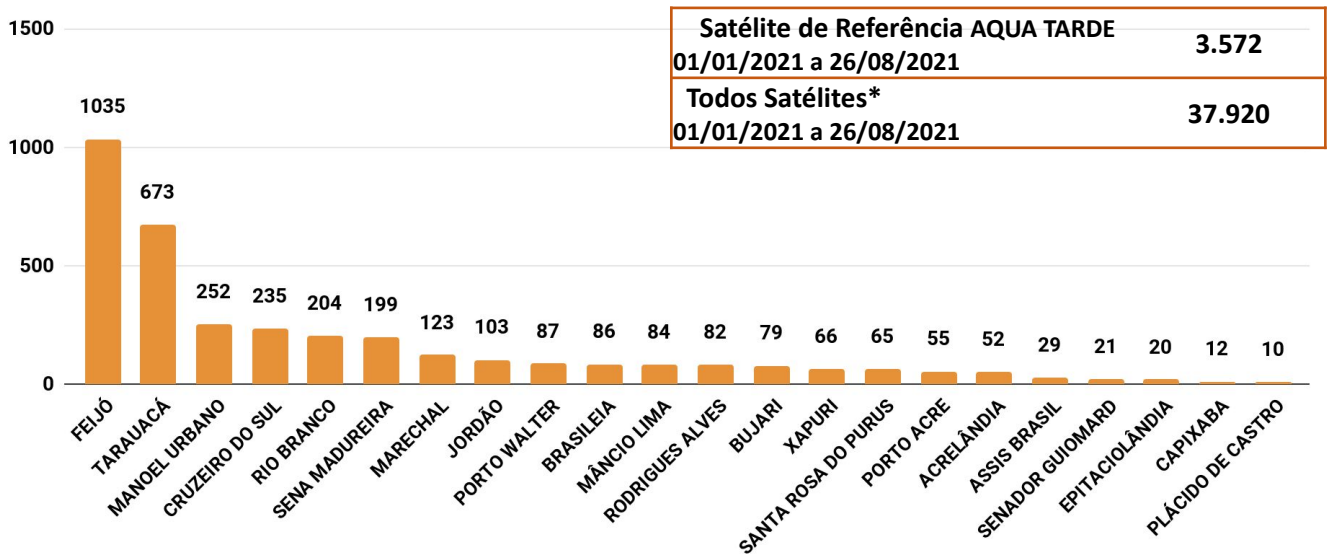
Figura 3 – Distribuição dos focos de queimadas acumulados de 01/01/2021 a 26/08/2021, no Estado do Acre. (Satélite de referência AQUA TARDE)
