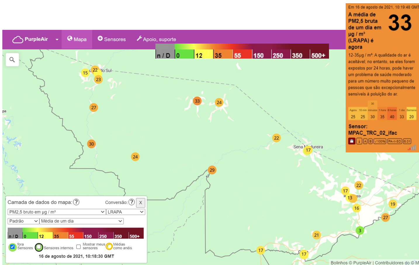
Figura 13 – Concentração de Material Particulado Raw PM 2.5 bruto \mu\text{g}/\text{m}^3 média para dia 16/08/2021
