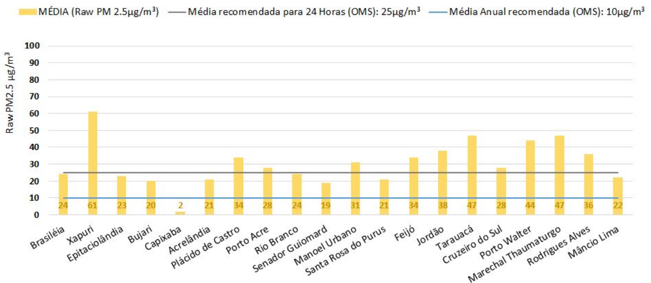
Rede de Monitoramento de Qualidade do Ar, Material Particulado Fino Raw PM2.5 \mu\text{g}/\text{m}^3 Dia: 15/08/2021 - Fonte: PurpleAir
